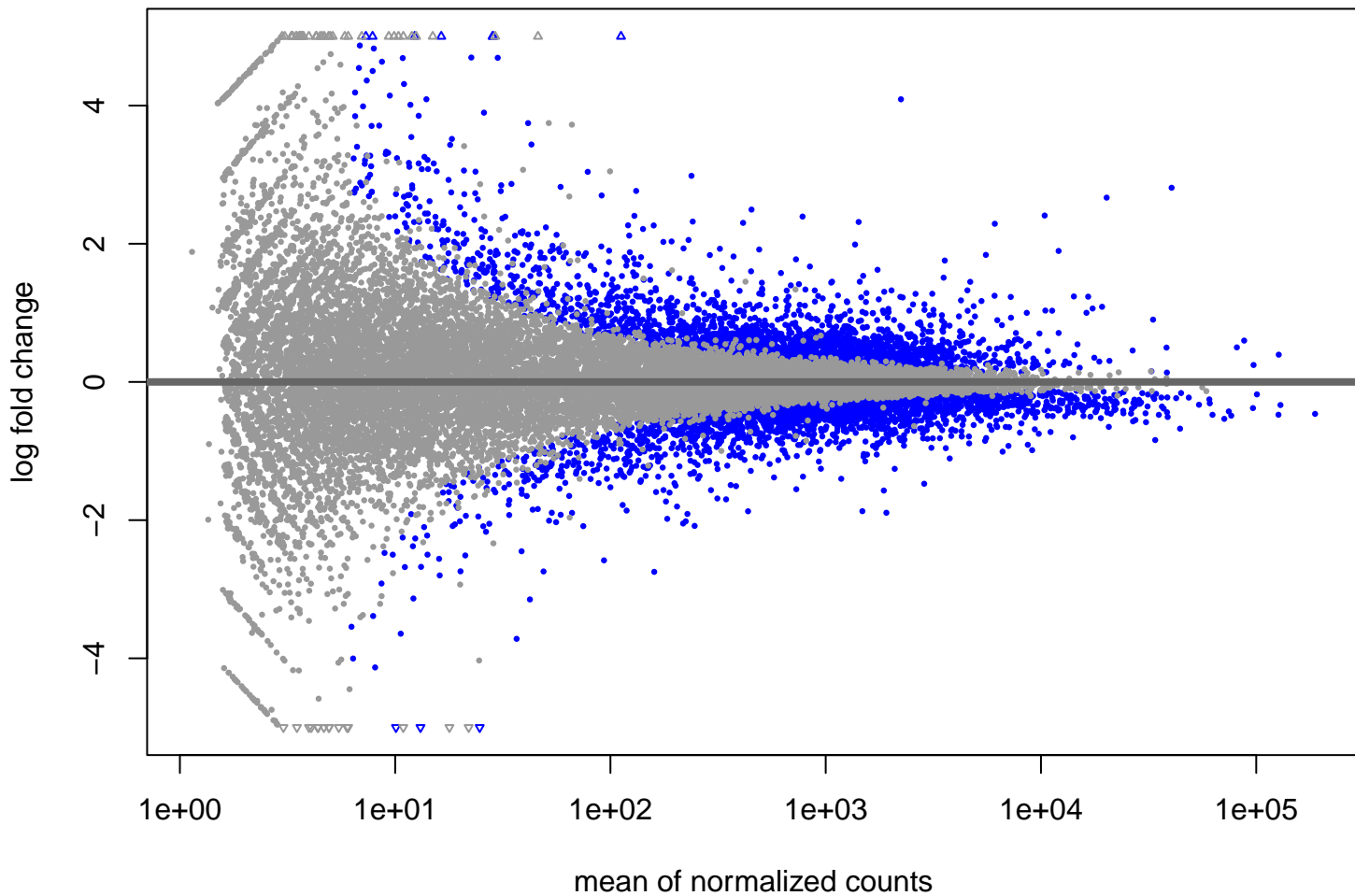
MA Plot: KO vs WT
