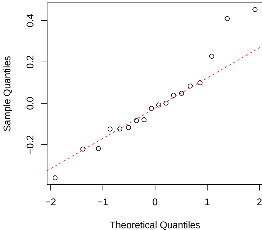
Narea | 3000 | Weinmannia Normal Q-Q
