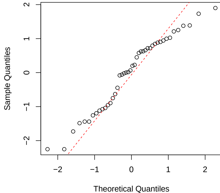
d13C | 2000 | Alchornea Normal Q-Q
