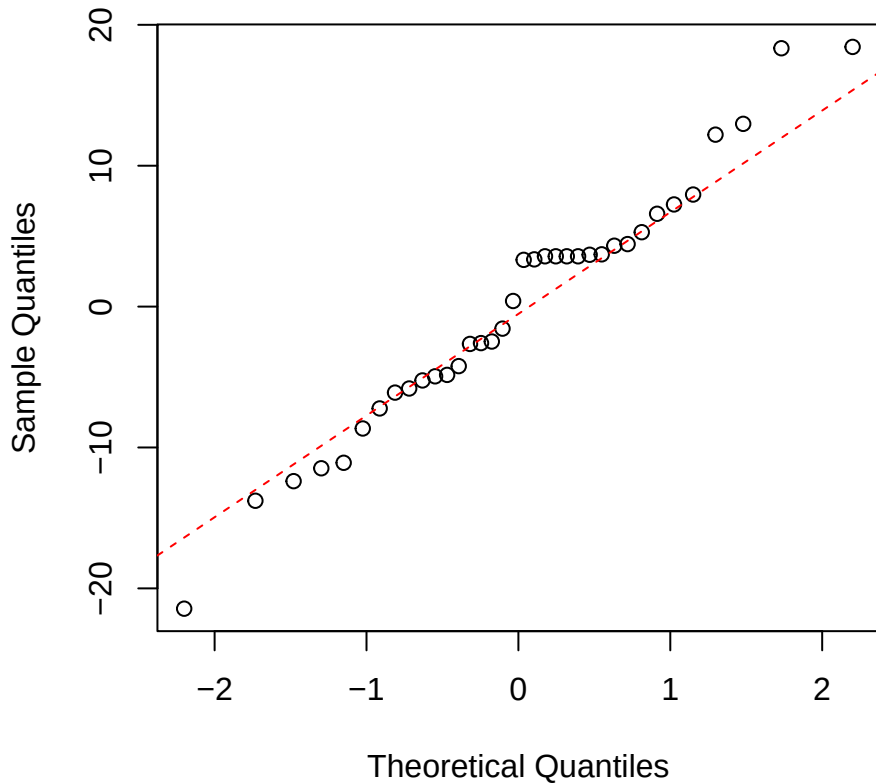
Carea | 1000 | Pouteria Normal Q-Q
