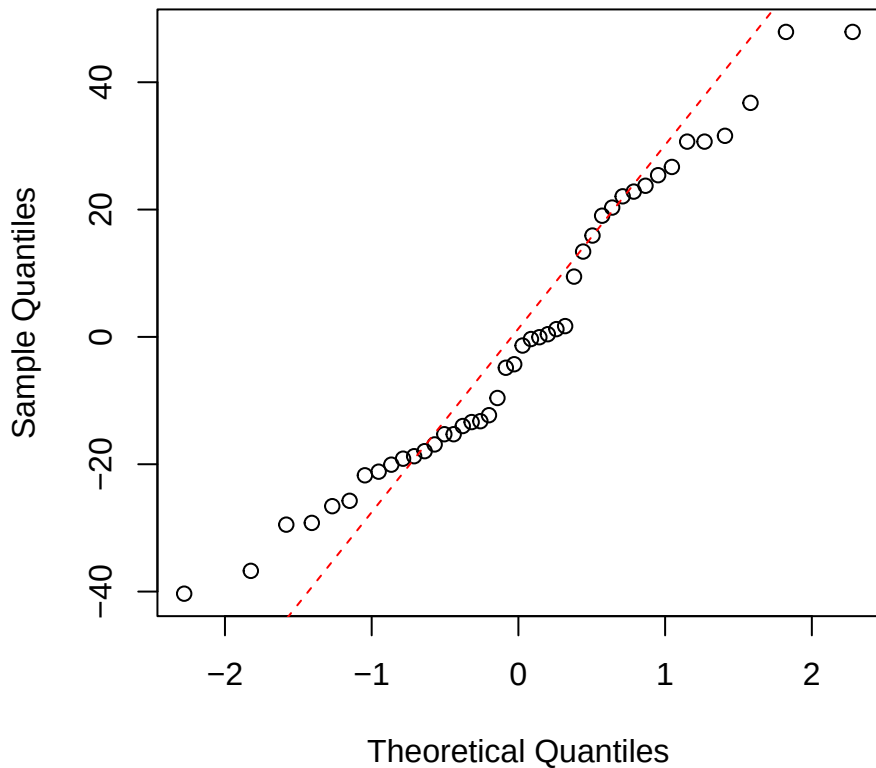
Ci | 2000 | Alchornea Normal Q-Q
