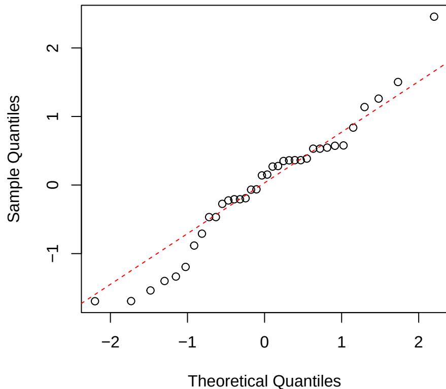
d13C | 1000 | Pouteria Normal Q-Q
