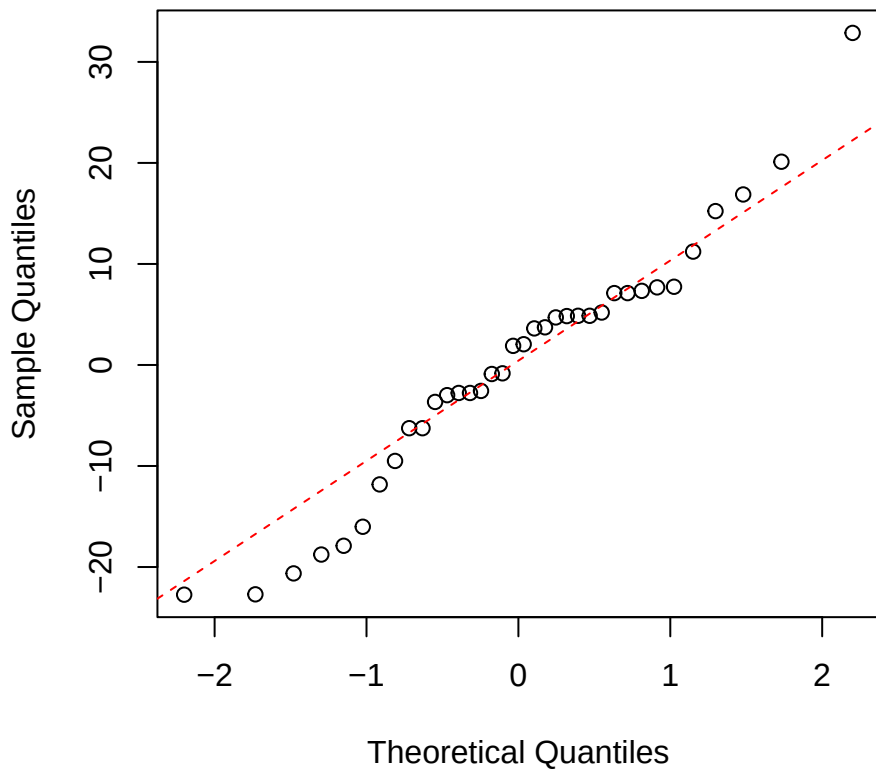
iWUE | 1000 | Pouteria Normal Q-Q
