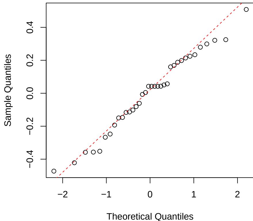
Narea | 1000 | Pouteria Normal Q-Q
