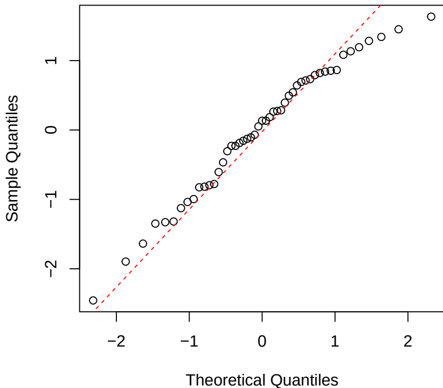
d13C | 2000 | Myrcia Normal Q-Q
