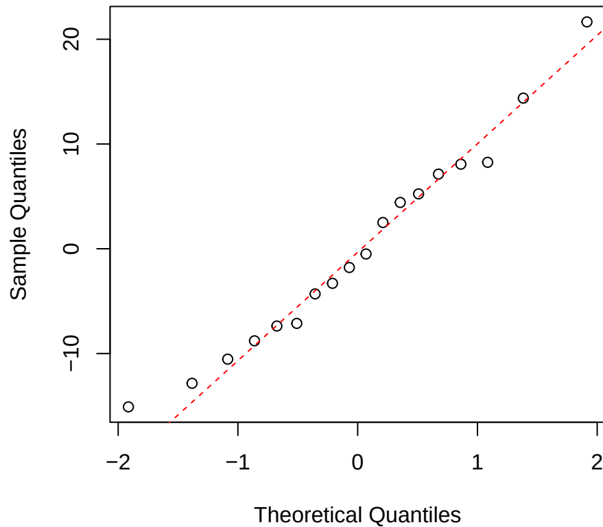
iWUE | 3000 | Weinmannia Normal Q-Q
