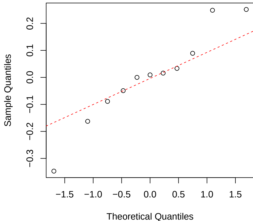
Narea | 1000 | Clarisia Normal Q-Q
