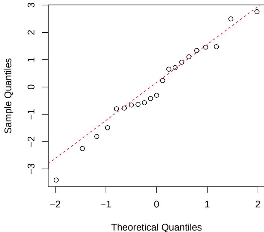
d13C | 3000 | Hedyosmum Normal Q-Q
