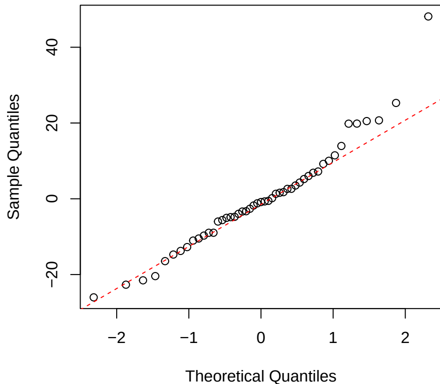
Carea | 2000 | Myrcia Normal Q-Q
