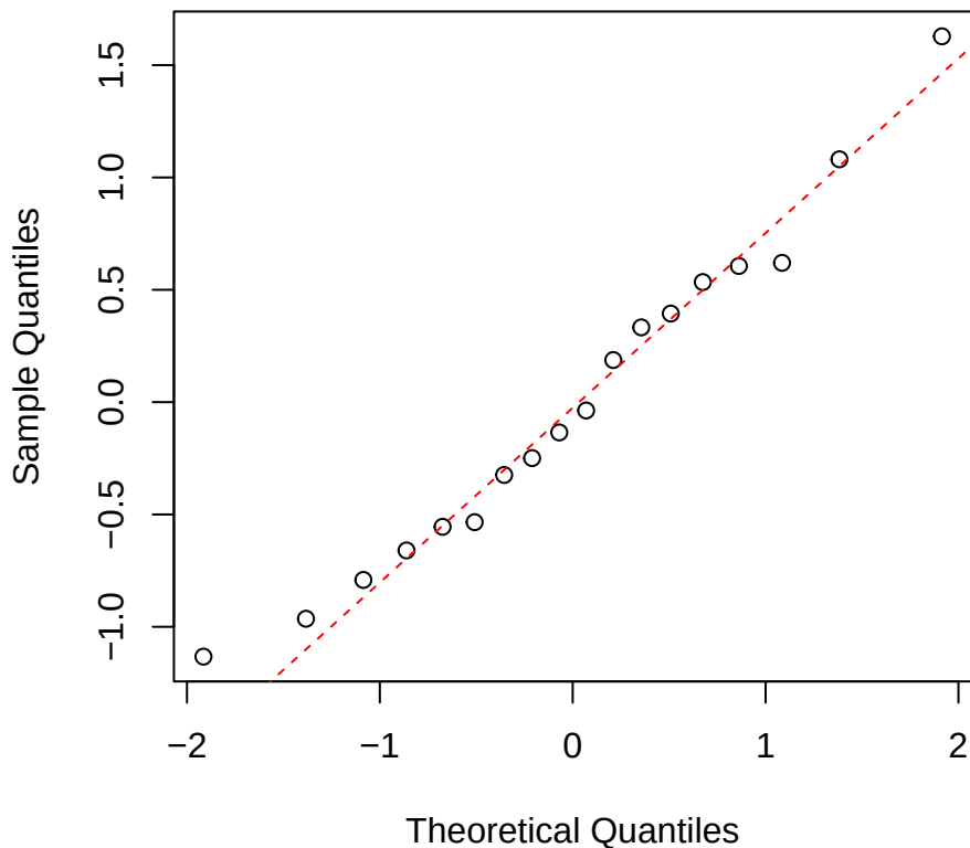
d13C | 3000 | Weinmannia Normal Q-Q
