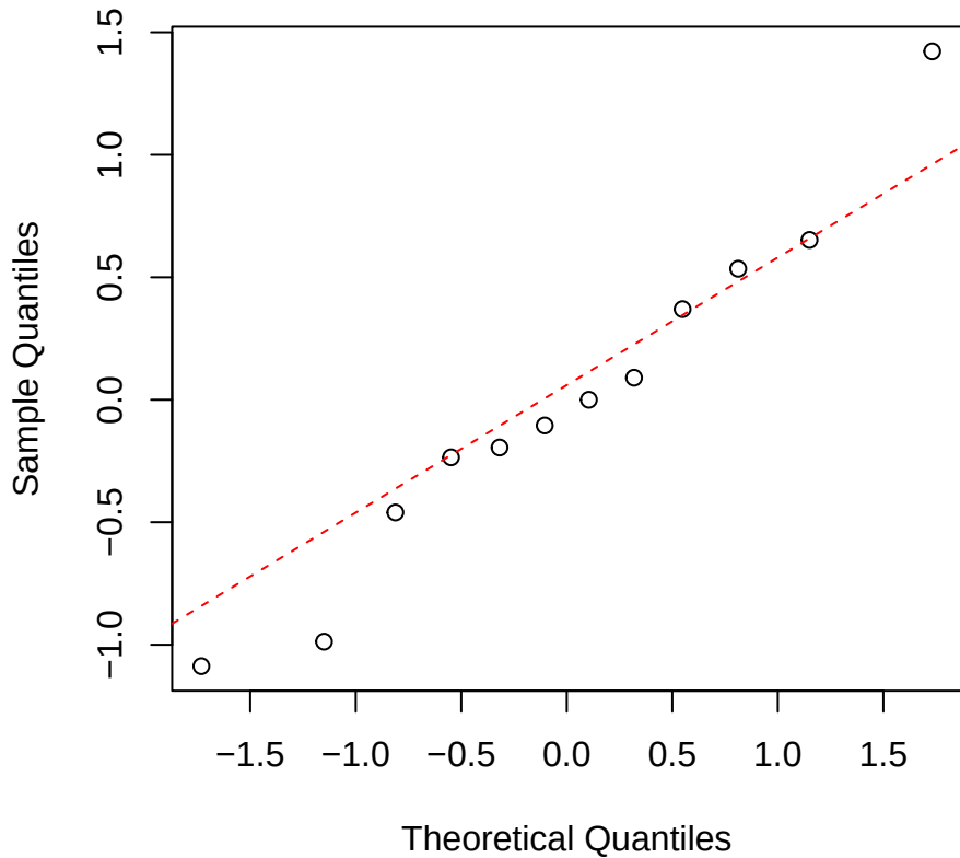
d13C | 1000 | Clarisia Normal Q-Q
