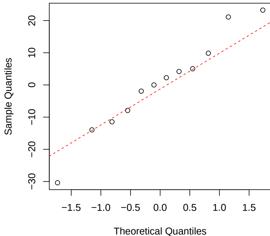
Ci | 1000 | Clarisia Normal Q-Q
