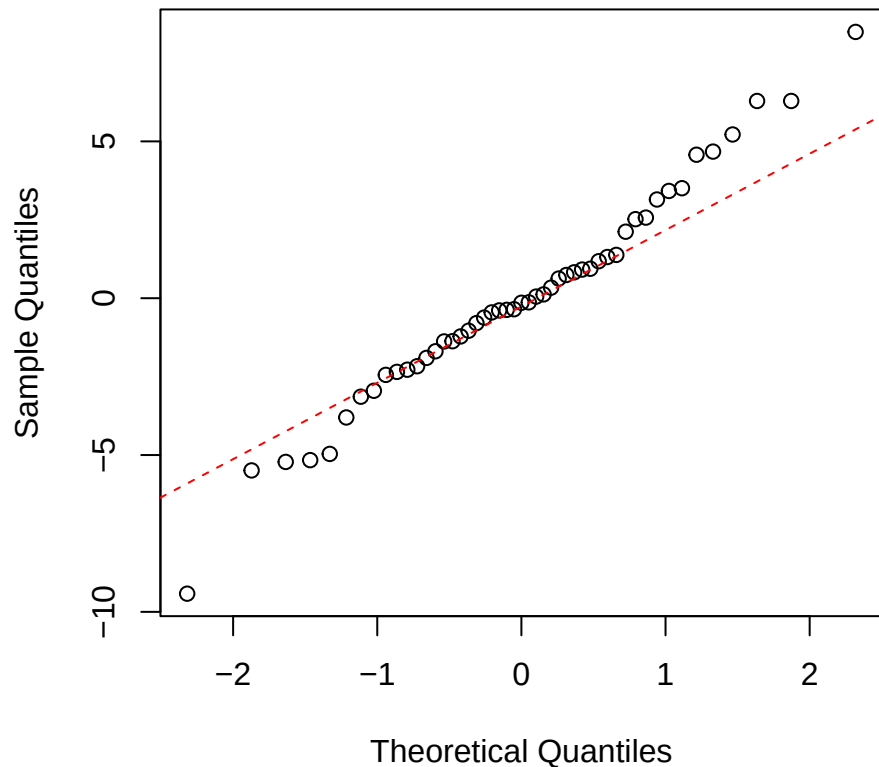
SLA | 2000 | Myrcia Normal Q-Q
