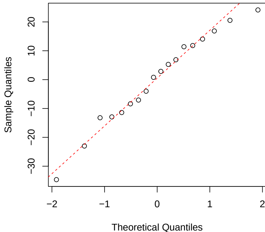
Ci | 3000 | Weinmannia Normal Q-Q
