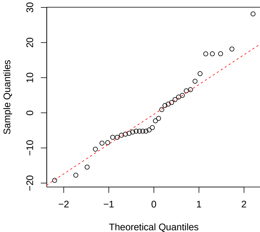
SLA | 1000 | Pouteria Normal Q-Q
