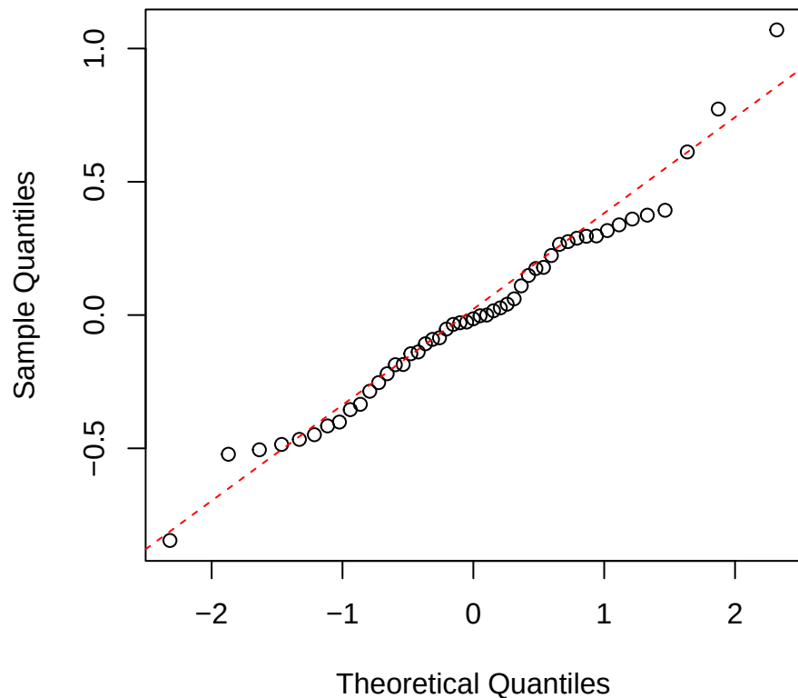
Narea | 2000 | Myrcia Normal Q-Q
