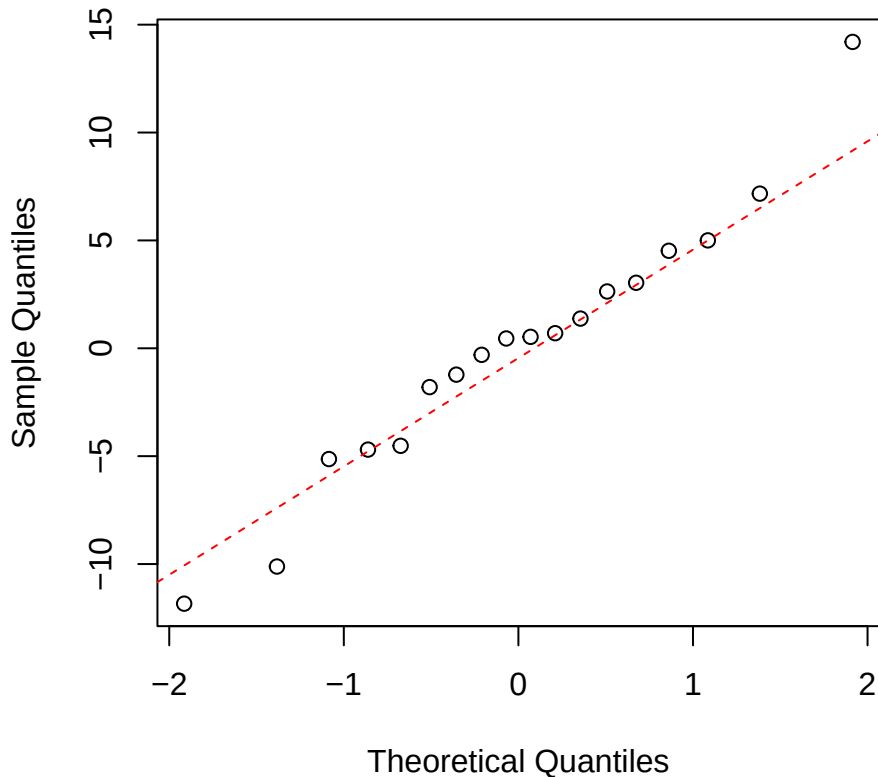
SLA | 3000 | Weinmannia Normal Q-Q
