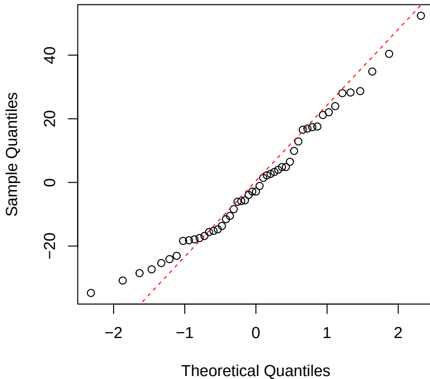
Ci | 2000 | Myrcia Normal Q-Q
