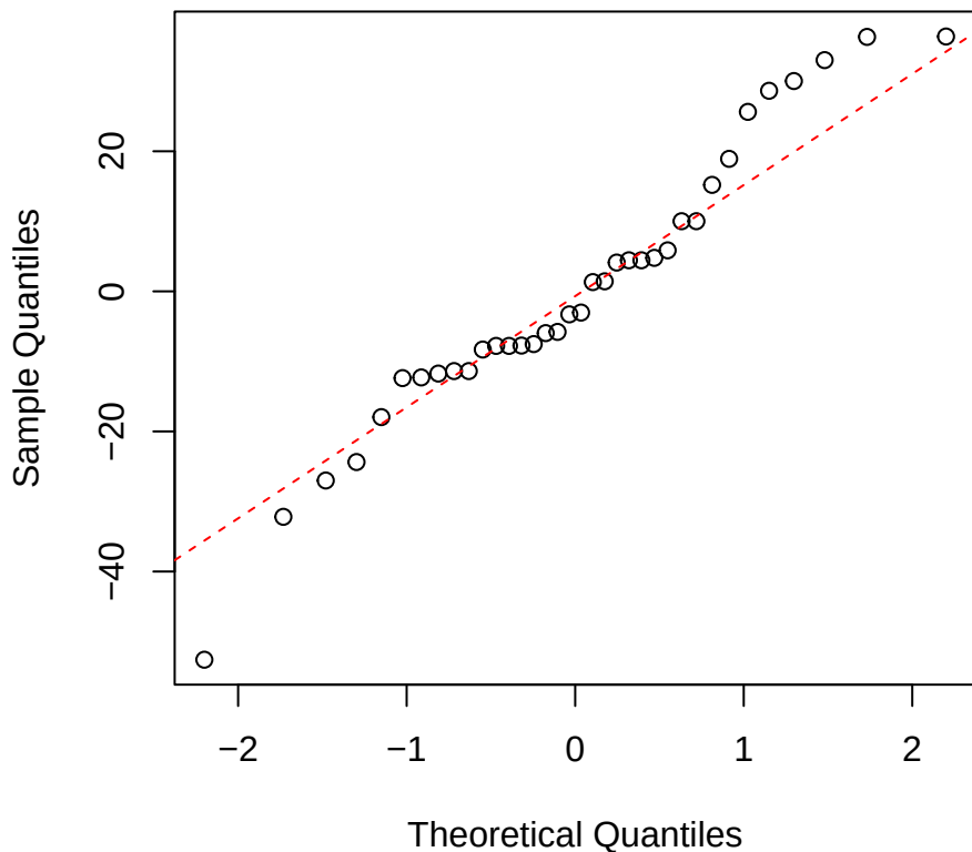
Ci | 1000 | Pouteria Normal Q-Q
