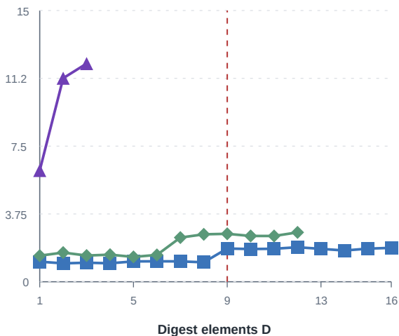
Verifier time (ms)
