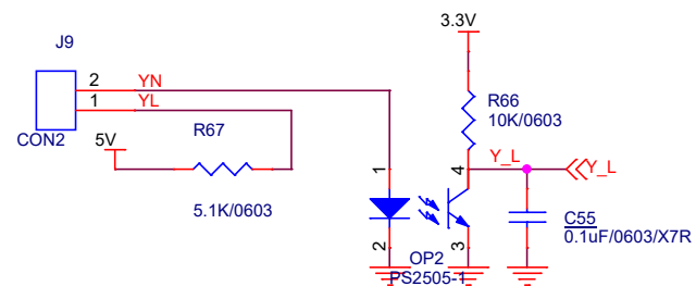
遥 信 监 测
