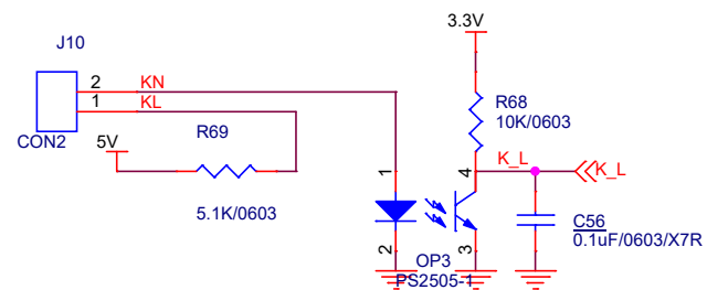
空 开 监 测
