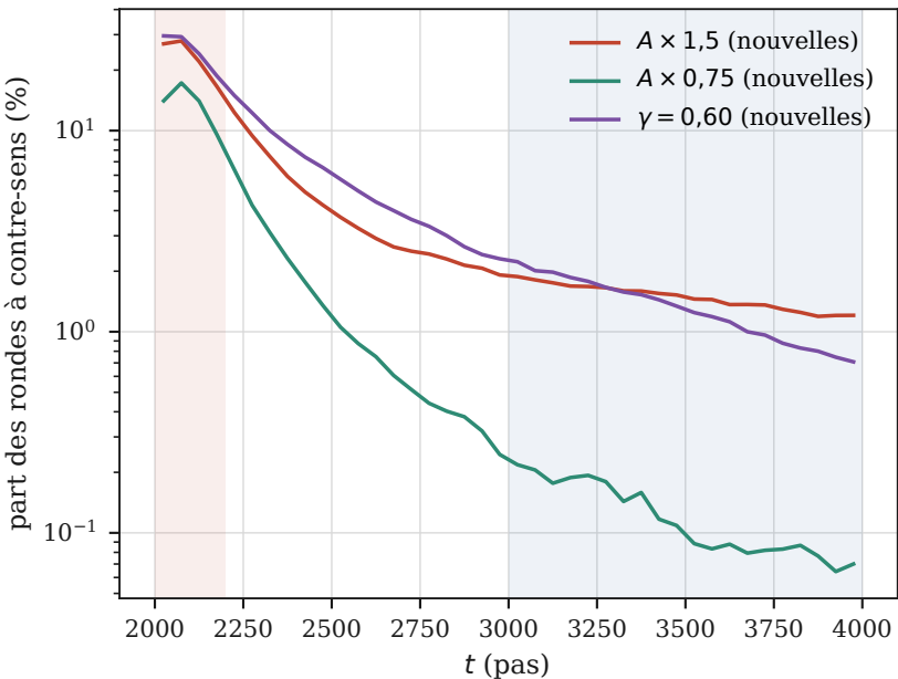
(a) moyenne sur douze graines, blocs de 50 pas
