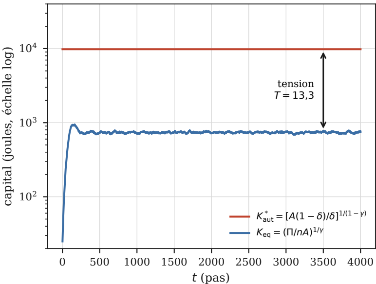
(a) les deux échelles que la tension compare
