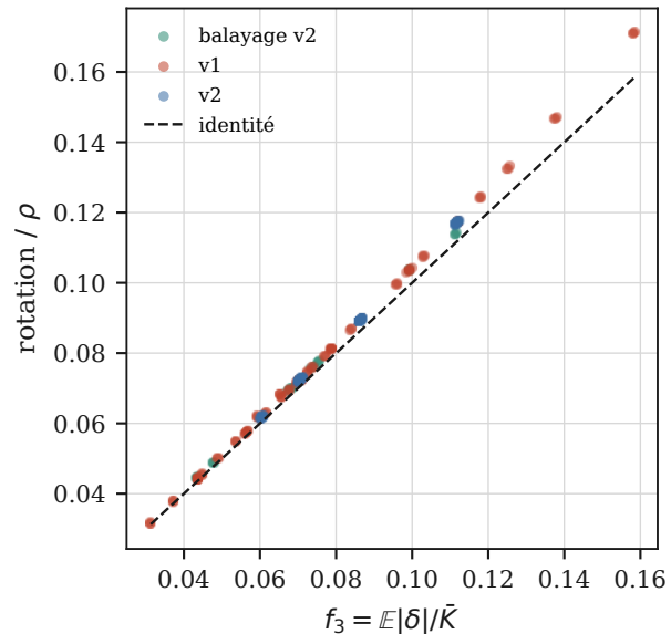
(c) toute la variation est dans f_3
