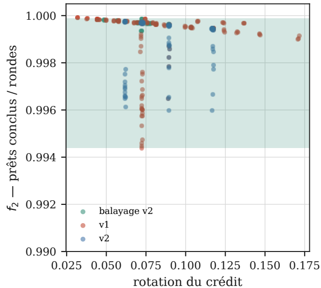
(b) f_2 — probabilité de traiter toute la plage : [0,9944 ; 0,9999]
