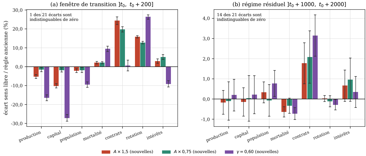
FIGURE 6 – Le levier agit fortement pendant la transition et presque plus après : c’est ce qui rend les deux fenêtres obligatoires. Écarts relatifs appariés par graine entre sens libre et règle ancienne, avec l’intervalle de Student à 5 % sur 12 – 1 degrés de liberté. Les deux échelles verticales ne sont pas les mêmes : le plus grand écart vaut 27,1 % à gauche et 3,1 % à droite. Ce qu’il faut regarder est le compte porté sur chaque panneau : sur les mêmes 21 écarts — sept observables \times trois bras — 1 seulement est indistinguishable de zéro pendant la transition, contre 14 dans le régime résiduel. Une lecture moyennée sur les mille pas aurait donné le panneau de droite, et conclu « pas d’effet ».
