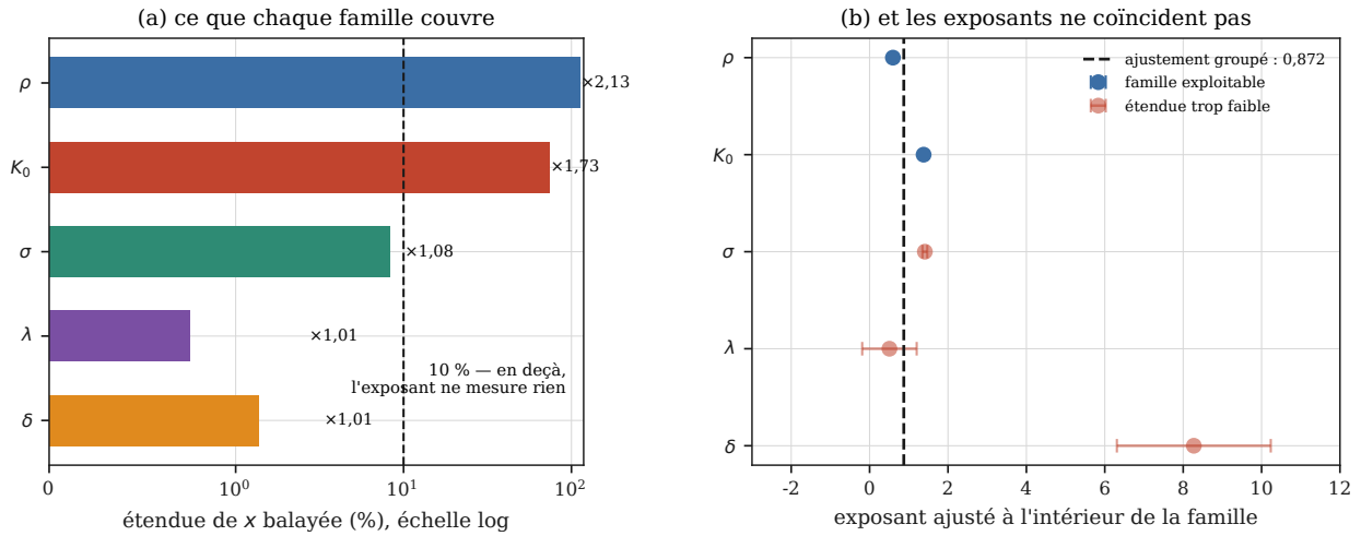
FIGURE 18 – Trois familles sur cinq ne couvrent pas assez de terrain pour que leur exposant veuille dire quoi que ce soit. À gauche, l'étendue de x que chaque famille balaie, en échelle logarithmique, avec le repère à 10 %. À droite, l'exposant ajusté à l'intérieur de chaque famille, avec son intervalle de Student, et le trait vertical de l'ajustement groupé. Ce qu'il faut regarder est double : les deux familles exploitables ( \rho et K_0 ) donnent des exposants qui ne se recouvrent pas, et aucune ne recouvre le groupé ; et l'exposant de \delta , à 8,272 sur une étendue de \times 1,01 , est du bruit affiché comme une pente.
