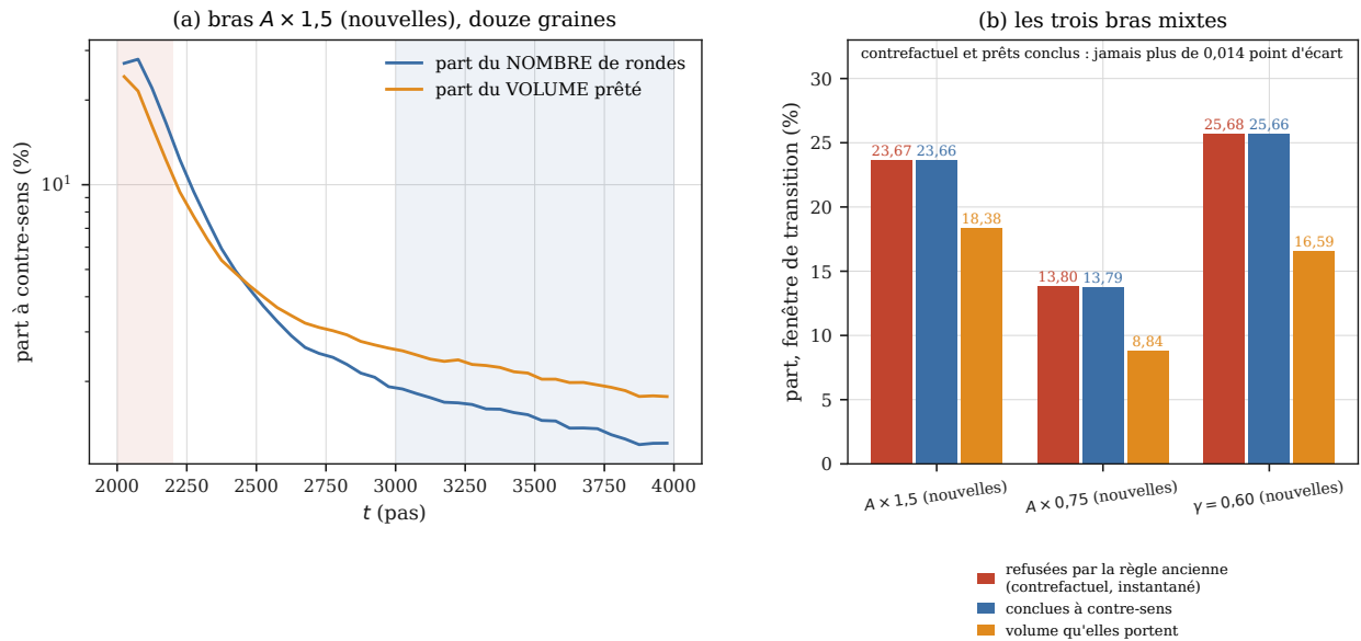
FIGURE 4 – Le nombre d'échanges à contre-sens et le volume qu'ils portent ne disent pas la même chose, et leur écart change de signe. À gauche, les deux parts sur toute la fenêtre. Ce qu'il faut regarder est le croisement : pendant la transition, les prêts à contre-sens sont plus petits que la moyenne — ils portent 18,38 % du volume pour 23,66 % des rondes — tandis qu'en régime résiduel ils sont plus gros . À droite, les trois bras mixtes dans la fenêtre de transition ; noter que le compteur contrefactuel (rouge) et les prêts effectivement conclus (bleu) ne s'écartent jamais de plus de 0,014 point de pourcentage, ce qui dit que presque toute paire refusée par l'ancienne règle conclut ici. (Les deux étiquettes de chaque paire de barres sont arrondies séparément : les soustraire donne jusqu'à deux centièmes, l'écart mesuré est plus petit.)
