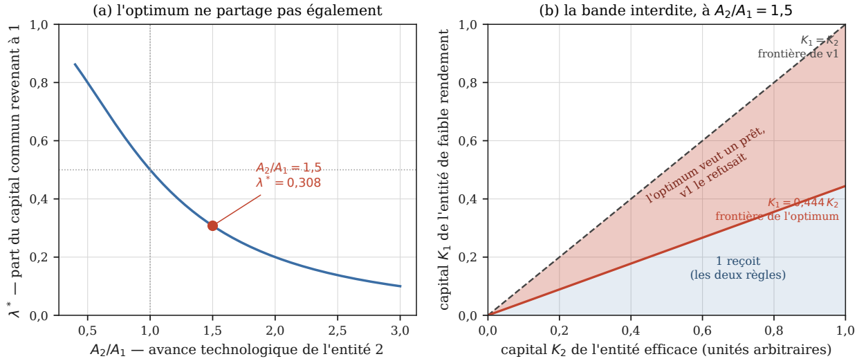
FIGURE 1 – Ce que la règle « la plus riche prête » s'interdisait n'est pas un cas limite : c'est une bande entière du plan des capitaux. À gauche, la part \lambda^* du capital commun que l'optimum laisse à l'entité la moins efficace ; elle vaut 1/2 quand les deux technologies coïncident et tombe à 0,308 dès que l'autre est une fois et demie plus productive. À droite, ce que cela donne dans le plan (K_1, K_2) : l'optimum demande à l'entité de faible rendement de céder dès que K_1 > 0,444 K_2 , là où l'ancienne règle ne l'autorisait qu'au delà de K_1 > K_2 . Regarder la largeur de la bande rouge — c'est exactement l'ensemble des paires que ce chantier débloque, et le §4 le retrouve en fréquence mesurée.
