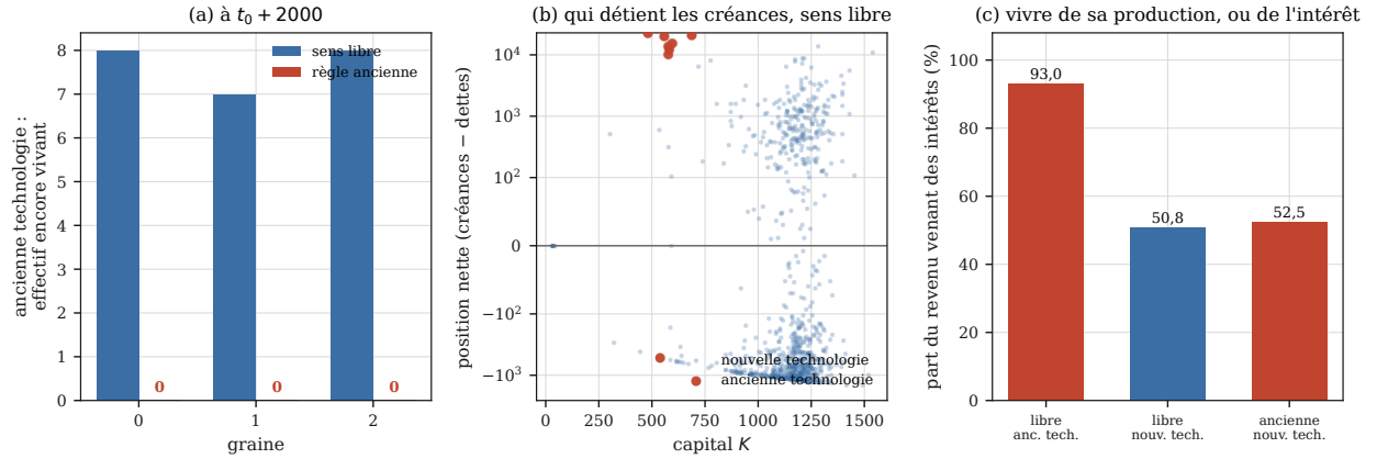
FIGURE 5 – Les survivantes de l'ancienne technologie ne produisent presque plus : elles vivent de l'intérêt. État entité par entité à t_0 + 2000 , bras new_A150 . À gauche, l'effectif survivant de la cohorte d'origine, graine par graine : sous l'ancienne règle il est nul sur les trois graines rejouées, et le zéro est écrit pour qu'on ne le confonde pas avec une donnée manquante. Au centre, ce qu'il faut regarder : les quelques points de l'ancienne technologie sont hauts et à gauche — position nette très positive, capital modeste — alors que le nuage de la technologie dominante est bas et à droite. À droite, la part du revenu qui vient des intérêts plutôt que de la production propre. Le rejeu qui produit cette figure reproduit la trajectoire de la campagne colonne par colonne, ce qui est vérifié avant de lire l'état final.
