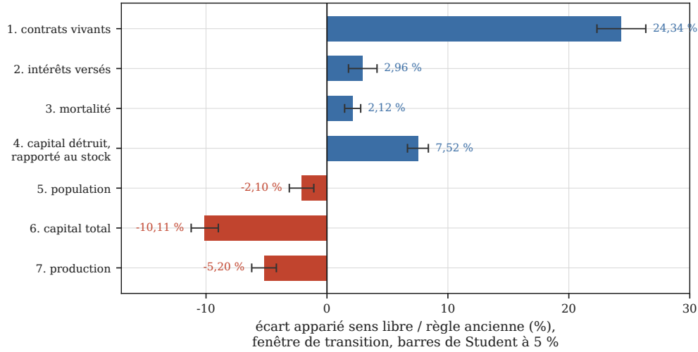
FIGURE 8 – Chaque maillon de la chaîne est mesuré et apparié, et le dernier a le signe opposé au premier. Écarts appariés entre sens libre et règle ancienne dans la fenêtre de transition, bras new_A150 , barres de Student à 5 %. Se lit de haut en bas : plus de contrats, donc plus de service perpétuel, donc plus de faillites, donc davantage de capital détruit par unité de stock , donc moins d'entités, moins de capital et moins de production. Le quatrième maillon est rapporté en part du stock et non en flux brut : le flux brut de capital détruit baisse de -3,35 %, parce que le stock dont il est tiré a baissé davantage, et le lire ainsi inverserait la conclusion.
