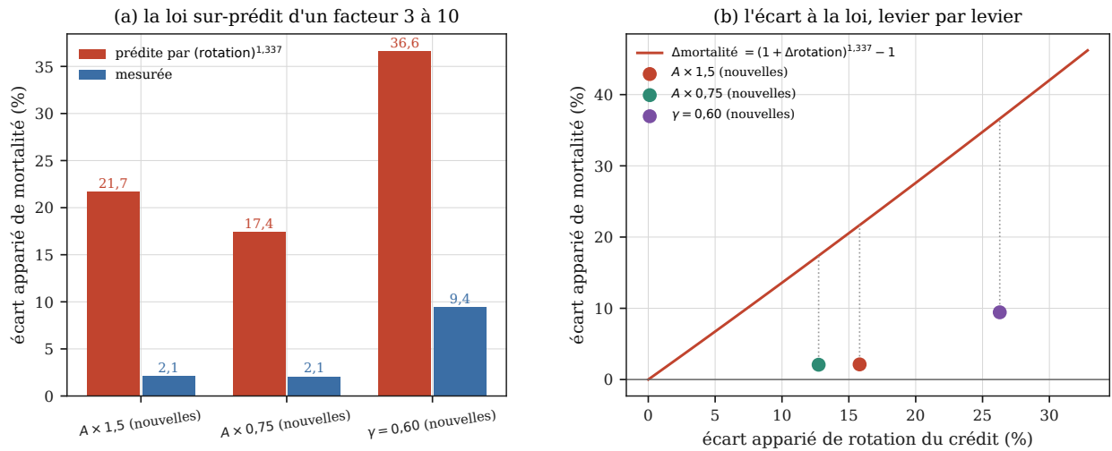
FIGURE 9 – La régularité de la lignée précédente ne range pas le cinquième levier. À gauche, pour chaque bras mixte, la hausse de mortalité que la loi (rotation) 1,337 prédit depuis la hausse de rotation mesurée, et celle qu'on mesure effectivement. À droite, les mêmes trois bras placés dans le plan de la loi, avec la courbe elle-même : ce qu'il faut regarder est la longueur des segments pointillés, qui est l'écart à la loi. [Incertitude] Cette fenêtre n'est pas un régime stationnaire, et la loi est une relation d'état stationnaire — le §4.6 dit pourquoi ce n'est pas encore une réfutation.
