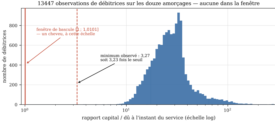
FIGURE 10 – La fenêtre de bascule est vide, et la figure dit de combien. Distribution du rapport capital / dû à l'instant du service, sur les 13 447 observations de débitrices des 12 amorçages, en échelle logarithmique. La bande rouge est la fenêtre [1 ; 1,0101] dans laquelle une débitrice basculerait ; le trait tireté marque le minimum observé. Ce qu'il faut regarder est la distance entre les deux — un facteur 3,2325 — et le fait que la distribution entière est à droite. Cette lecture précède le lancement du bras traité : c'est une prédiction, pas un constat.
