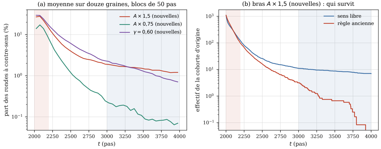
FIGURE 3 – Le régime nouveau ne s'éteint pas : il plafonne, et c'est une poignée de survivantes qui le tient. À gauche, la part des rondes concluant un prêt à contre-sens, moyennée sur 12 graines et par blocs de 50 pas, en échelle logarithmique. Regarder la forme : une décroissance rapide, puis un palier net — alors que la cohorte d'origine n'est pas renouvelée et que sa durée de vie moyenne est de trente-quatre pas. À droite, l'explication : sous le sens libre, l'effectif de cette cohorte cesse de décroître et se stabilise ; sous l'ancienne règle il va à l'extinction. Les deux fenêtres de lecture sont ombrées, en rouge la transition et en bleu le régime résiduel.
