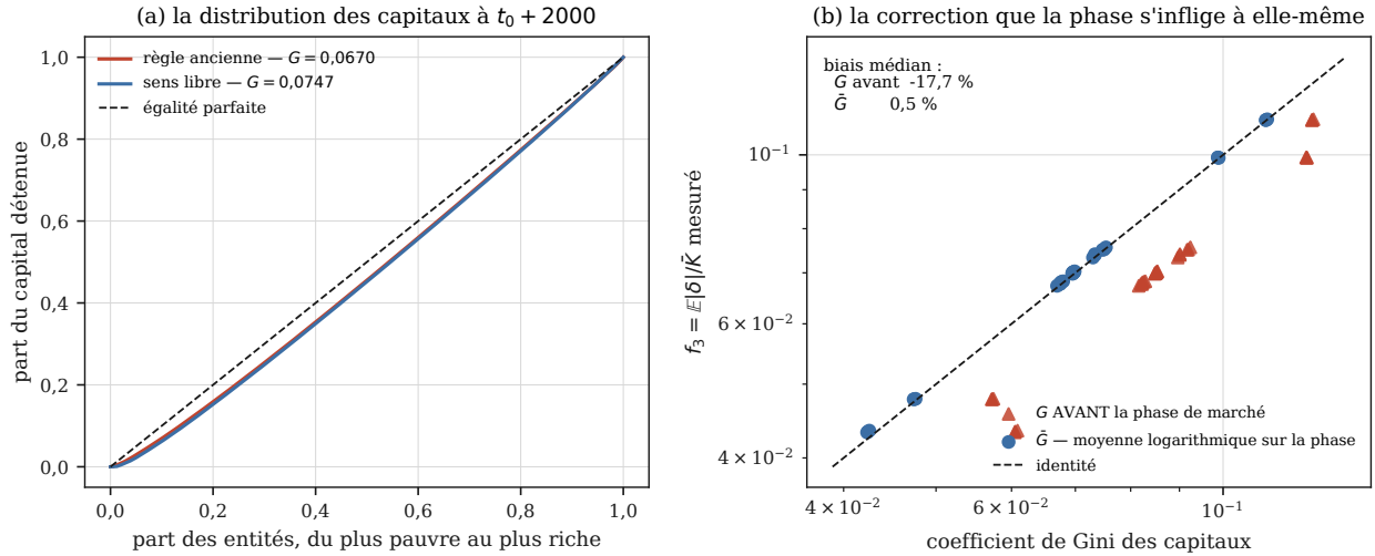
FIGURE 15 – La phase de marché resserre la distribution qu’elle consomme, et l’ignorer fausse la relation de dix-sept pour cent. À gauche, la courbe de Lorenz des capitaux à t_0 + 2000 sous les deux règles : elle donne au coefficient de Gini le sens qu’un nombre seul ne donne pas — l’aire entre la courbe et la diagonale, doublée. À droite, ce qui est réellement mesuré : f_3 contre le Gini pris avant la phase de marché (triangles) et contre sa moyenne logarithmique sur la phase (disques). Ce qu’il faut regarder est de quel côté de la diagonale tombent les triangles — le Gini d’avant surestime systématiquement — et à quel point les disques s’y recollent.
