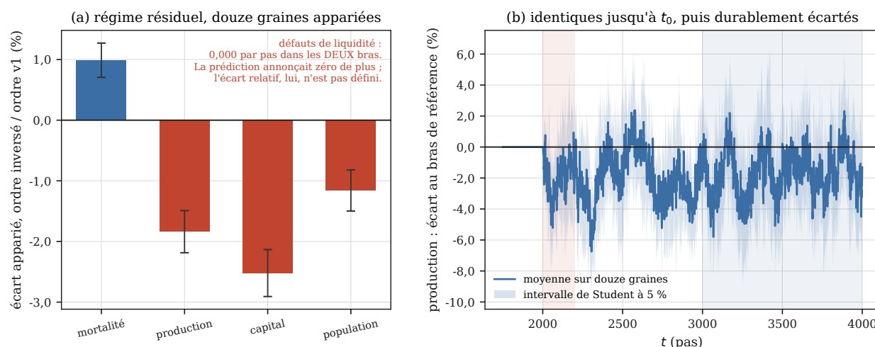
FIGURE 11 – Aucun défaut de plus, et pourtant des agrégats déplacés de plusieurs pour cent. À gauche, les écarts appariés sur le régime résiduel avec leurs barres de Student : la première colonne, celle des défauts de liquidité, est exactement nulle — c'est ce que la prédiction annonçait. À droite, l'écart de production au bras de référence, pas par pas : les deux bras sont rigoureusement identiques jusqu'à t_0 puisqu'ils partagent leur amorçage, puis s'écartent et restent écartés. C'est la marque d'un mécanisme qui ne crée pas d'événement mais déplace un flux à chaque pas.
