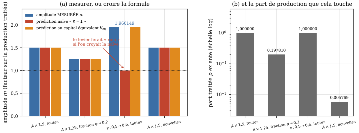
FIGURE 13 – Un levier sur l'exposant n'est pas un cadran de puissance : son amplitude dépend du capital. À gauche, pour chacun des quatre leviers, l'amplitude mesurée par le moteur au pas où l'intervention agit, la prédiction naïve qu'on ferait en supposant K = 1 , et la prédiction faite au capital équivalent. Ce qu'il faut regarder est la troisième colonne : la prédiction naïve annonce que le levier sur \gamma ne fait rien ( m = 1,000000 ), et la mesure donne 1,960149. À droite, la part de production que chaque levier touche ex ante , en échelle logarithmique : trois ordres de grandeur séparent une portée « toutes » d'une portée « nouvelles ».
