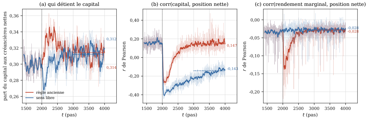
FIGURE 7 – La signature du changement de règle est un changement de signe , pas de niveau . Trois diagnostics sur un run apparié (bras new_A150 , graine 0) ; trait clair, la valeur pas à pas, trait épais, sa moyenne glissante sur 25 pas. Le trait vertical marque t_0 , les segments pointillés le niveau moyen du régime résiduel. Ce qu'il faut regarder est le panneau central : la corrélation entre capital et position nette reste positive sous l'ancienne règle (+0,147) et devient négative sous le sens libre (-0,143). À gauche, la part du capital détenue par les créancières nettes, elle, ne bouge presque pas : ce n'est pas la quantité de capital prêté qui change, c'est qui le prête.
