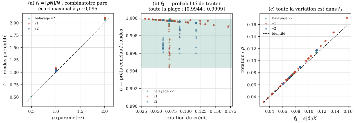
FIGURE 14 – Deux facteurs sur trois sont pinés, et le troisième porte toute la variation. Les trois facteurs de (11) sur 322 runs des deux lignes. À gauche, f_1 suit \rho à la partie entière près. Au centre, f_2 ne quitte jamais la bande verte, large de six millièmes : presque toutes les paires tirées traitent. À droite, la rotation divisée par \rho se confond avec f_3 sur la diagonale. Ce qu'il faut regarder est l' absence de dispersion dans les deux premiers panneaux comparée au troisième — c'est ce qui autorise à ne plus étudier que f_3 .
