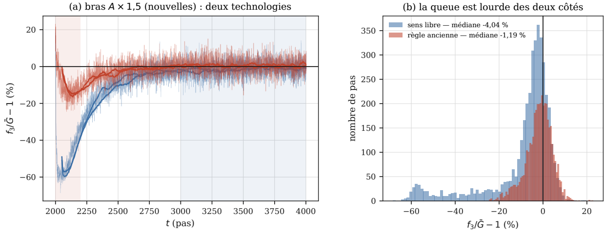
FIGURE 16 – Hors du régime homogène la relation reste bonne en médiane, mais elle se trompe de moitié pendant les épisodes les plus pondérés. Écart relatif entre f_3 mesuré et \bar{G} , pas par pas, sur le bras new_A150 où deux technologies coexistent ; trait clair, la valeur pas à pas, trait épais, sa moyenne glissante. Les deux fenêtres de lecture sont ombrées. À droite, la distribution des mêmes écarts. Ce qu'il faut regarder est l'asymétrie : la masse est contre zéro, et la queue part vers les écarts négatifs — f_3 tombe sous \bar{G} quand le rééquilibrage est le plus fortement pondéré, c'est-à-dire pendant la transition.
