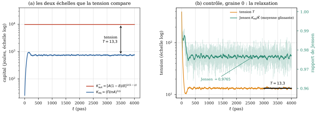
FIGURE 12 – La tension est le rapport de deux échelles, et le calcul natif rend le second terme exact. À gauche, l'échelle autarcique K_{\text{aut}}^* — constante, elle ne dépend que de A , \delta et \gamma — et le capital équivalent K_{\text{eq}} , qui monte pendant la relaxation puis se stabilise ; la flèche est la tension. À droite, sa décroissance, et le rapport de Jensen K_{\text{eq}}/\bar{K} sur l'axe de droite. Ce qu'il faut regarder est que le rapport de Jensen s'écarte de 1 de plus de deux pour cent : c'est l'écart que la reconstruction a posteriori de la lignée précédente devait estimer, et que le calcul dans le moteur donne exactement, ses deux termes étant pris au même instant du pas.
