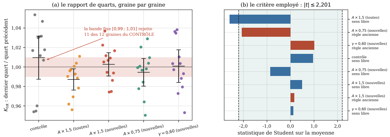
FIGURE 2 – Un seuil hérité d'une autre fenêtre ne mesurerait ici que la longueur de la fenêtre. À gauche, le rapport de quarts sur K_{\text{tot}} , graine par graine, avec la moyenne et son intervalle de Student ; la bande rouge est le seuil fixe [0,99 ; 1,01] hérité de la lignée précédente. Regarder la colonne du contrôle — un bras qui ne subit aucune intervention et dont on sait qu'il est stationnaire : 11 de ses 12 graines tombent hors de la bande. À droite, le critère effectivement employé, qui teste la moyenne du rapport contre 1 ; la zone verte est la région d'acceptation.
