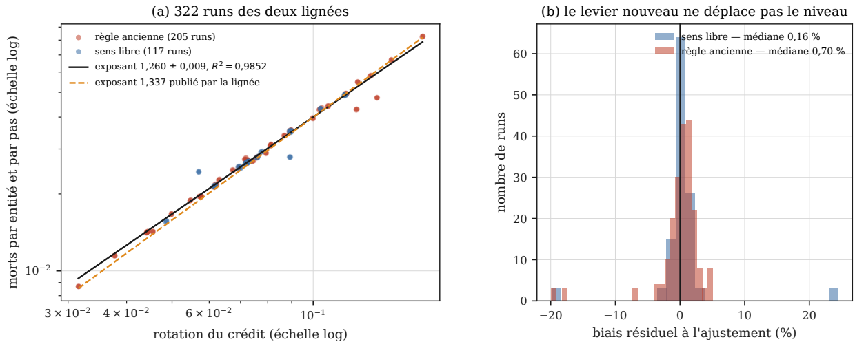
FIGURE 19 – Sur tout le corpus des deux lignées, la mortalité suit la rotation sur une plage d’un facteur cinq. À gauche, les 322 runs en échelle logarithmique, colorés par règle de sens, avec l’ajustement groupé et, en tireté, l’exposant 1,337 publié par la lignée précédente. Ce qu’il faut regarder est que les deux règles s’interpénètrent : un run à sens libre tombe sur la même courbe qu’un run à règle ancienne. À droite, le biais résiduel à l’ajustement, par règle. [Incertitude] Le corpus mélange les deux lignées, les deux règles et des transitoires ; l’exposant qui en sort décrit une population plus hétérogène que les 109 runs sur lesquels le 1,337 a été publié, et les deux ne sont pas directement comparables.
