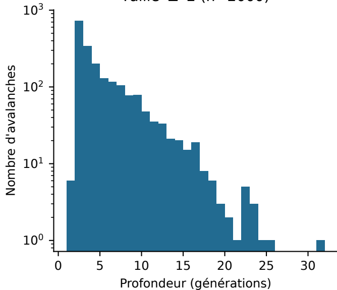
Taille \geq 2 (n=2000)
