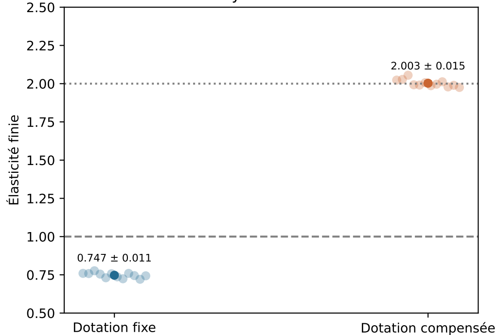
Mesure \neq symétrie de tout l'état
