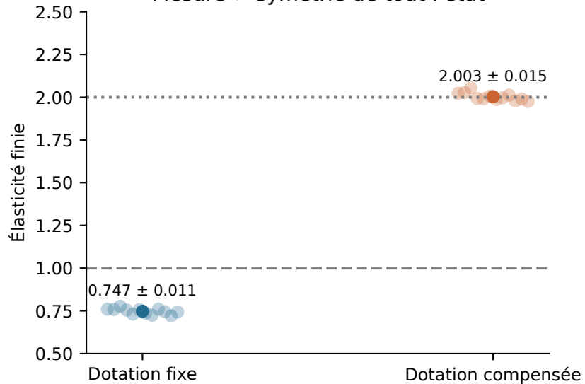
Mesure \neq symétrie de tout l'état
