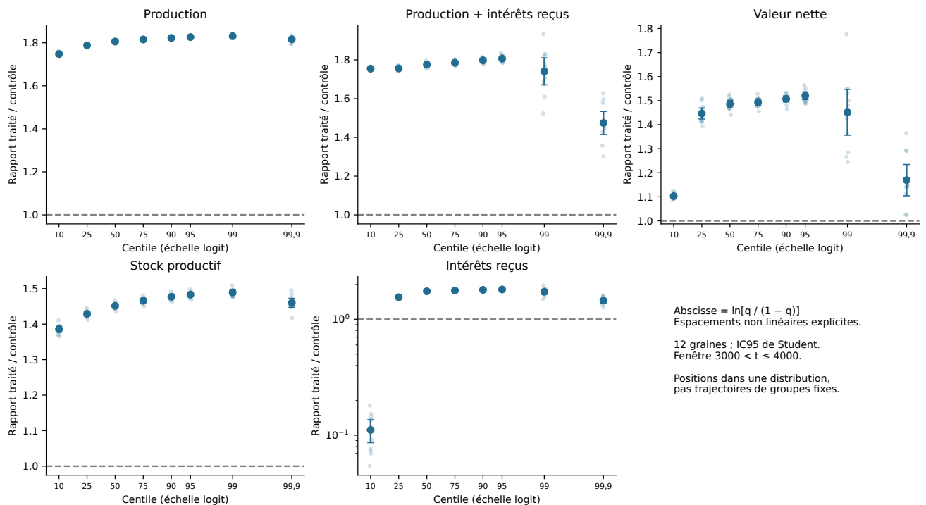
Figure 14 – Lire des positions, pas des groupes fixes. M4.4, A \times 1,5 à dotation fixe, douze graines, 3000 < t \leq 4000 . Les abscisses sont placées à \ln[q/(1-q)] , puis graduées en centiles : l'échelle non linéaire est explicite et laisse les quantiles extrêmes lisibles. Points pâles : rapports par graine ; points pleins et barres : moyenne et IC95. Une ordonnée 1,8 signifie que le quantile considéré vaut 1,8 fois celui du contrôle ; elle ne signifie pas que les mêmes entités ont gagné 80 %.
