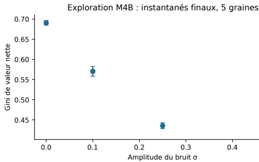
Figure 9 – Revenir aux leviers étudiés pendant la construction du modèle. Confirmation M4B, cinq graines indépendantes par cellule, T = 4000 . Gini de valeur nette calculé sur l'instantané final, non Gini du capital ni du bassin. Les autres paramètres sont ceux du centre historique M4B, notamment k = 3 ; seul \sigma varie. Le balayage ancien de k n'est pas représenté ici, les expériences principales ultérieures fixant les rencontres à deux entités. Les barres sont des IC95 de Student recalculés depuis les valeurs par graine.
