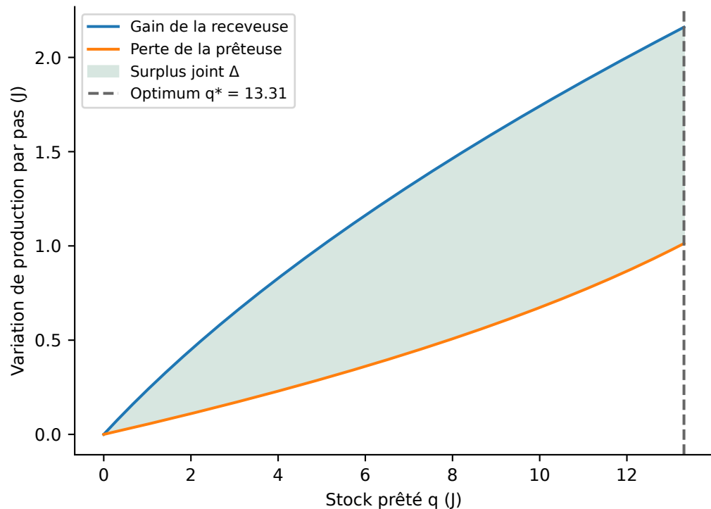
Transfert de 1 vers 2, jusqu'à l'optimum
