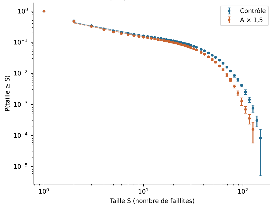
Survie empirique et tendance sur 2 \leq S \leq 30
