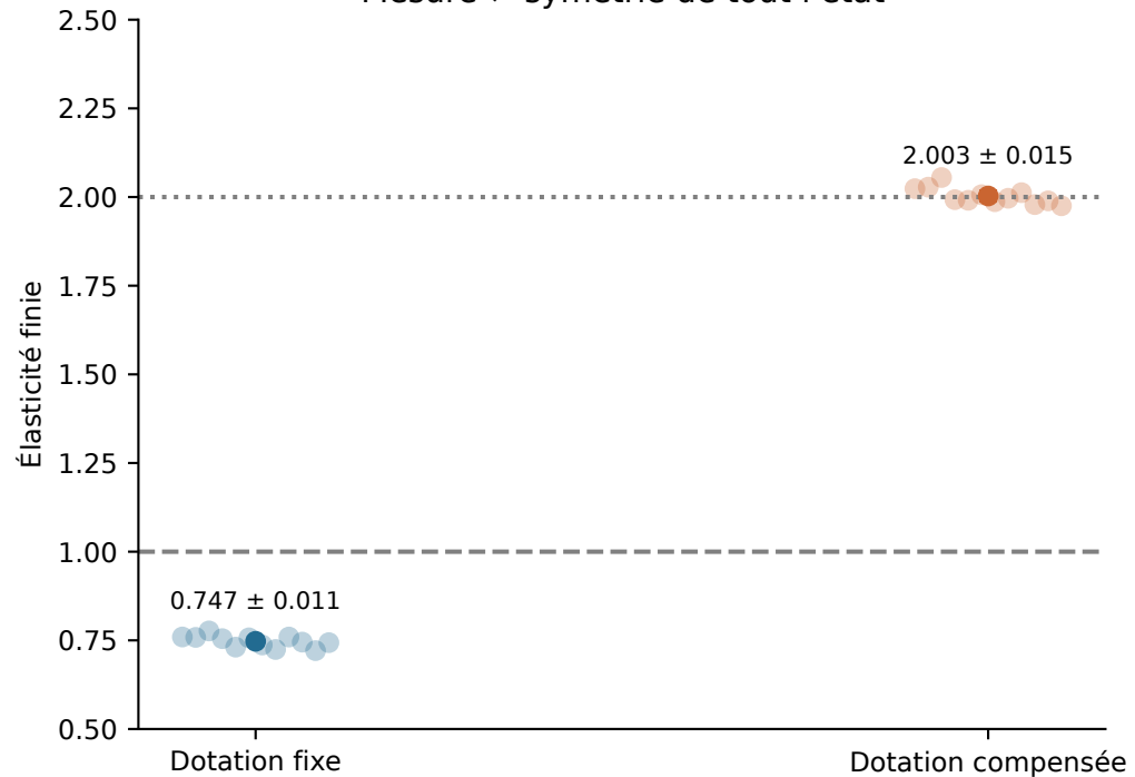
Mesure \neq symétrie de tout l'état
