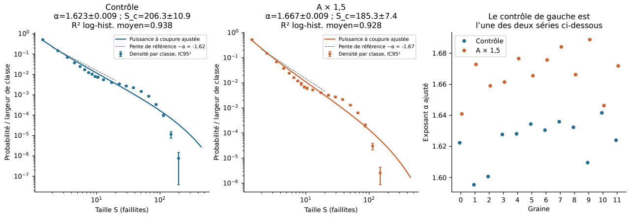
Figure 4 – Histogrammes, ajustements et répétitions. M4.4, douze graines par condition, 3000 < t \leq 4000 . Les points donnent la probabilité par classe divisée par la largeur de classe ; les barres sont des IC95 inter-graines. Les courbes sont les moyennes des ajustements discrets à coupure exponentielle, les rubans un bootstrap de 2000 tirages de runs entiers. Les droites tiretées indiquent la pente -\alpha de référence, pas la loi tronquée complète. Les R^2 sont calculés sur les logarithmes des classes non vides, puis moyennés entre graines. Le panneau gauche représente le contrôle dont les exposants individuels sont repris à droite ; le panneau central représente l'autre série. 1 Les barres trop longues pour l'échelle log sont tronquées à 95 % du niveau ; leurs valeurs intégrales restent dans les données.
