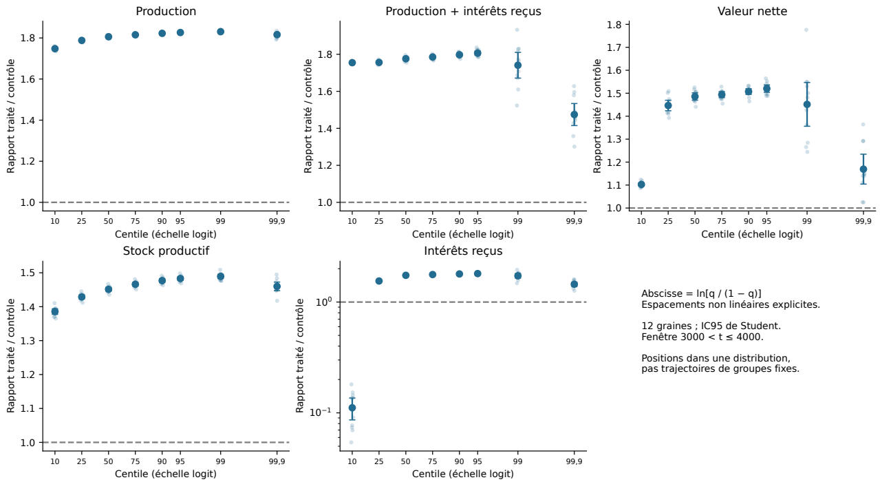
Figure 12 – Lire des positions, pas des groupes fixes. M4.4, A \times 1,5 à dotation fixe, douze graines, 3000 < t \leq 4000 . Les abscisses sont placées à \ln[q / (1 - q)] , puis graduées en centiles : l'échelle non linéaire est explicite et laisse les quantiles extrêmes lisibles. Points pâles : rapports par graine ; points pleins et barres : moyenne et IC95. Une ordonnée 1,8 signifie que le quantile considéré vaut 1,8 fois celui du contrôle ; elle ne signifie pas que les mêmes entités ont gagné 80 %.
