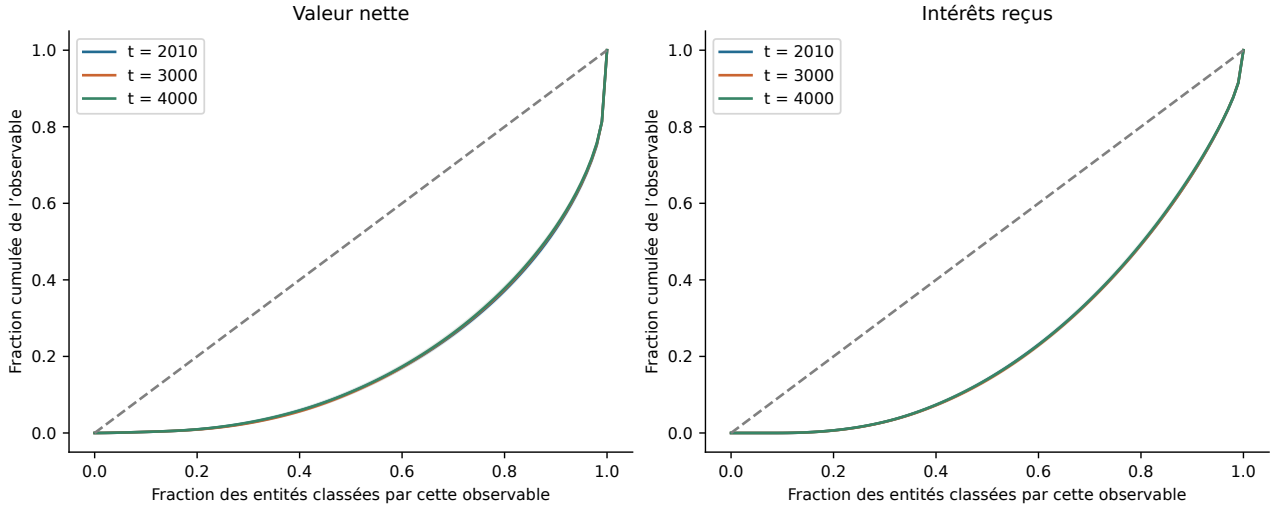
Figure 6 – La distribution collective persiste malgré le renouvellement individuel. Contrôle M4.4, douze graines : courbes de Lorenz à t = 2010, 3000 et 4000 , et IC95 inter-graines. Chaque observable possède son propre classement.
