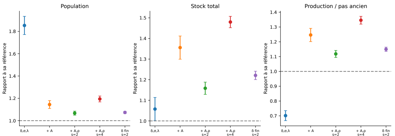
Figure 9 – Le changement de pas ne s'arrête pas à trois substitutions. Expériences Live-v1 depuis un état vide, trois graines par configuration. Fenêtre commune 1200 < t_{\text{ancien}} \leq 2000 . Les flux des pas regroupés sont divisés par s , pas les stocks. Les trois premiers essais regroupent deux pas ; le quatrième en regroupe quatre. Le dernier compare deux configurations à \delta = 0,002 avant conversion, et possède donc sa propre référence. Points : rapports par graine moyennés ; barres : IC95 de Student, larges avec trois répétitions.
