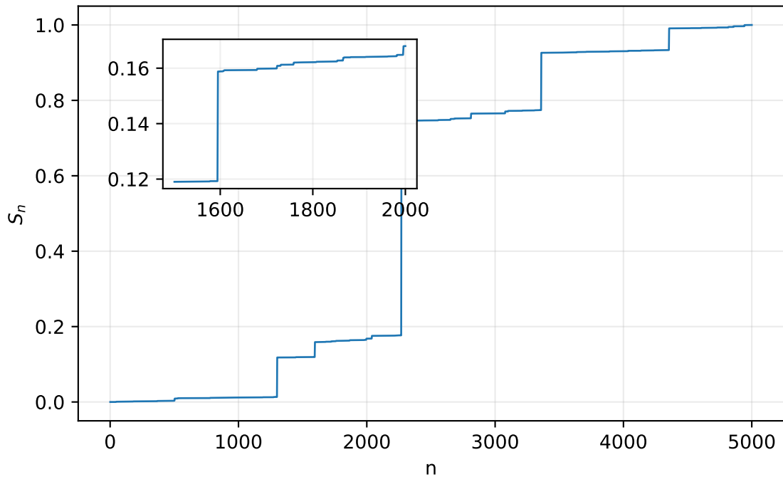
Pareto \mu = 0.5 , N=5000
