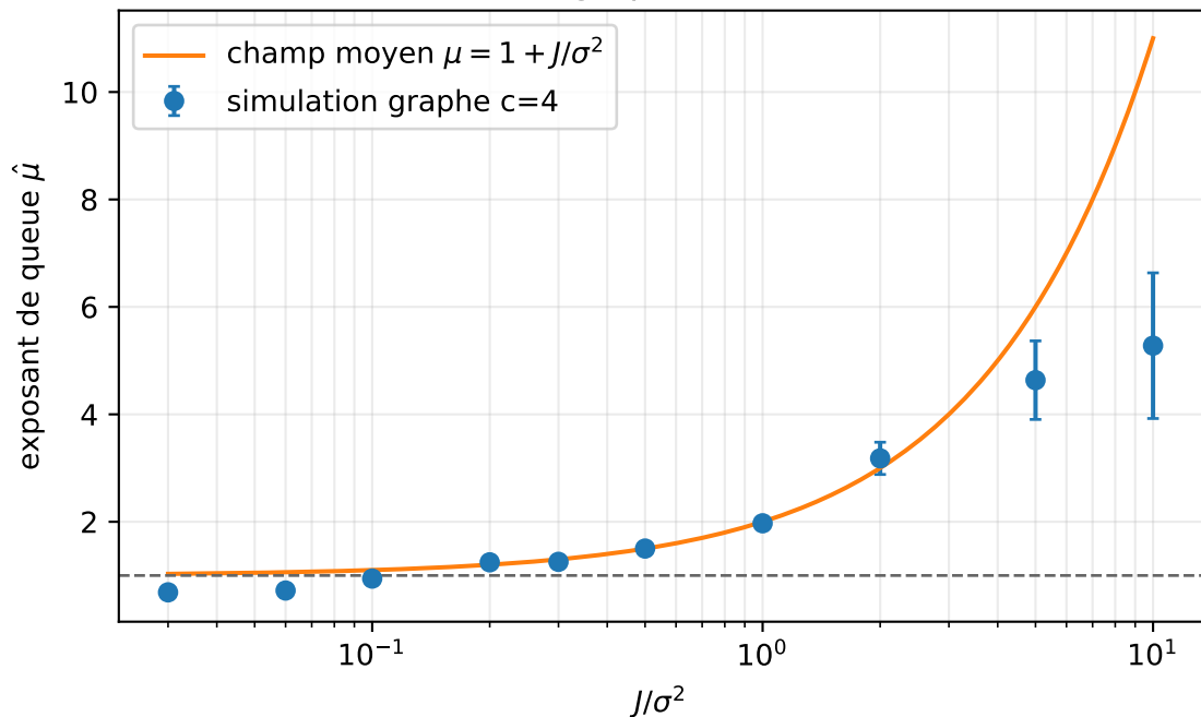
Modèle sur graphe aléatoire, c=4
