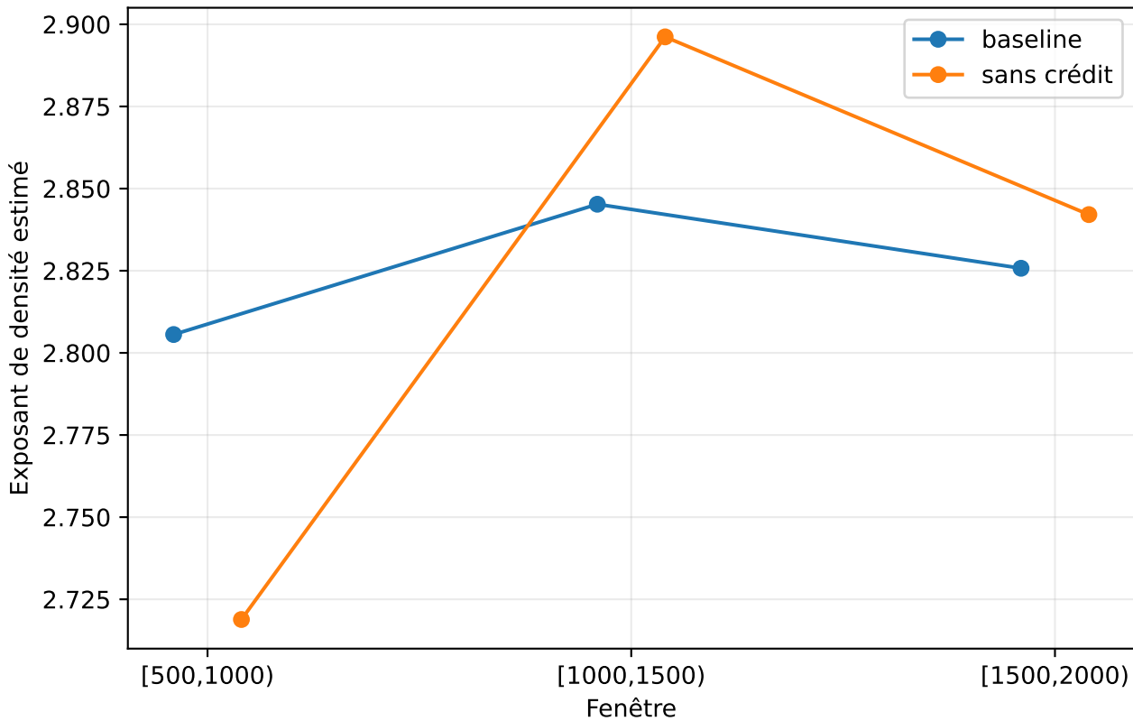
Queue de NW : baseline contre ablation sans crédit
