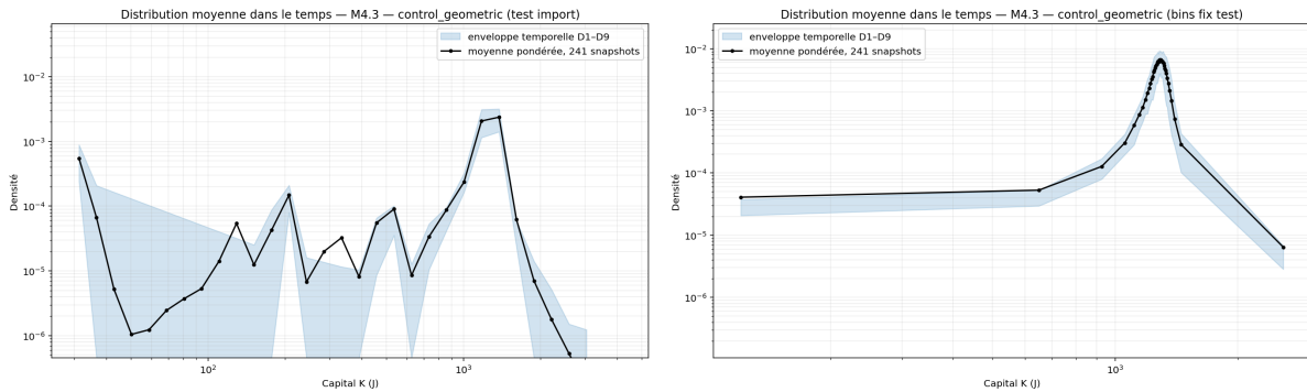
FIGURE 14 — entity_size_histo_temporal_mean.png , control_geometric/seed 0 , avant (gauche, bornes log uniformes) et après (droite, bornes aux quantiles) le correctif. Mêmes données, même fonction appelante — seul le choix des bornes change.
