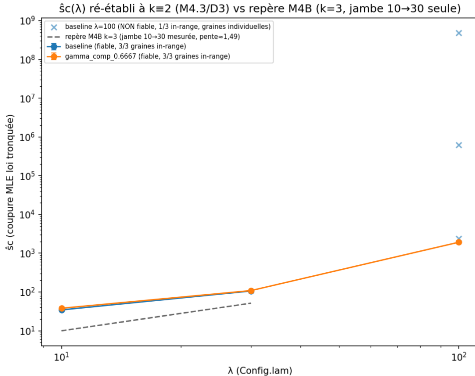
FIGURE 13 – \hat{s}_c(\lambda) ré-établi à k \equiv 2 (baseline et gamma_comp_0.6667 ) contre le repère M4B à k = 3 (jambe 10 → 30 seule, la seule mesurée par M4B). Points non fiables affichés individuellement (croix), pas de moyenne, pas de ligne les reliant aux points fiables.
