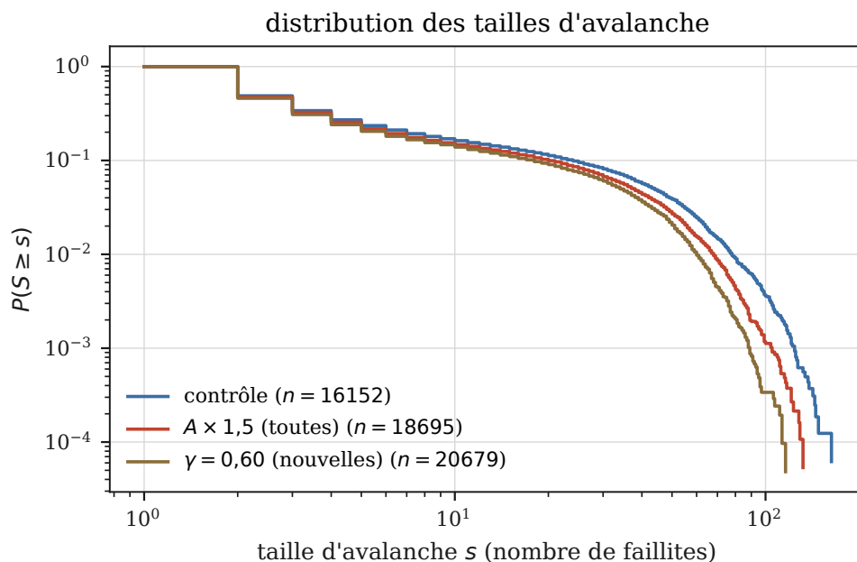
FIGURE 47 – Fonctions de survie d'avalanches par réalisation. Fonction de survie empirique, quatre graines par bras. La coupure de taille finie est visible au-delà de la centaine de faillites.
