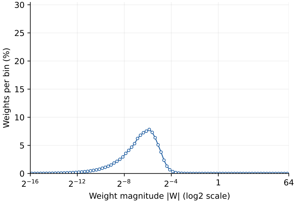
FP16
