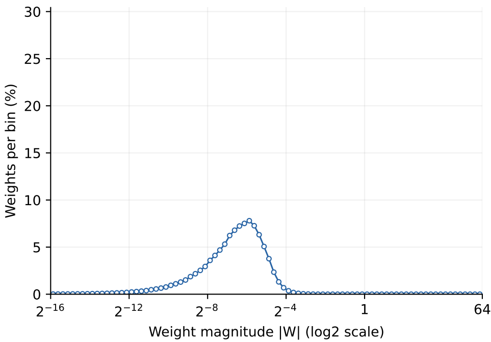
FP16
