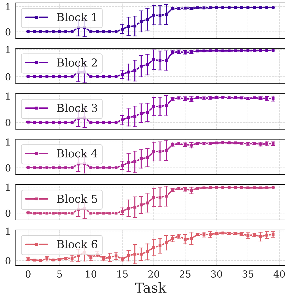
VIT Duplicate fraction
