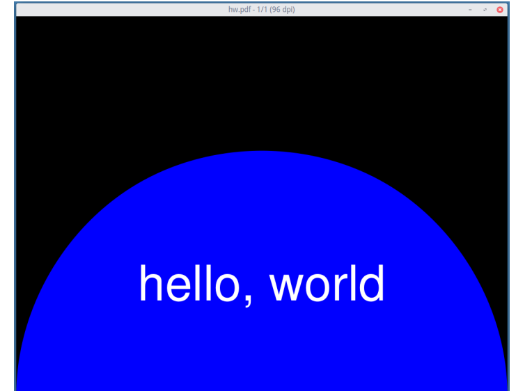
Linux: mupdf
