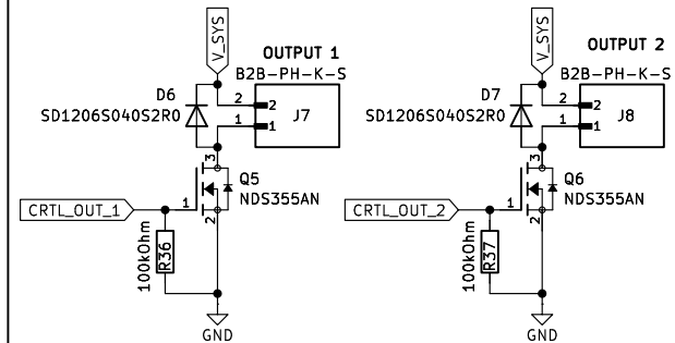
MOSFET OUTPUTS
