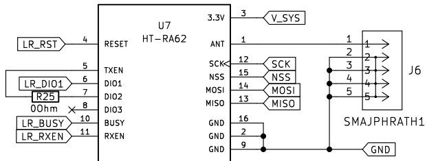
LORA MODULE HT-RA62
