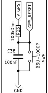
GPS RESET
