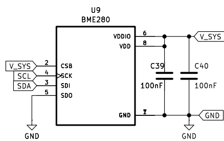
BME280 SENSOR
