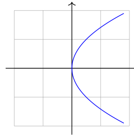
parabola
