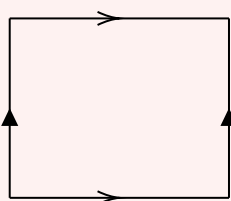
Subdivision of T^2
