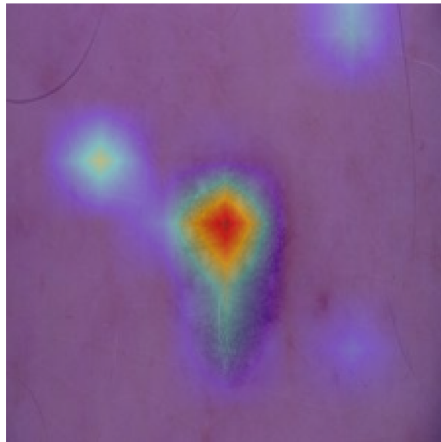
EfficientNetV2B0 P=0.197
