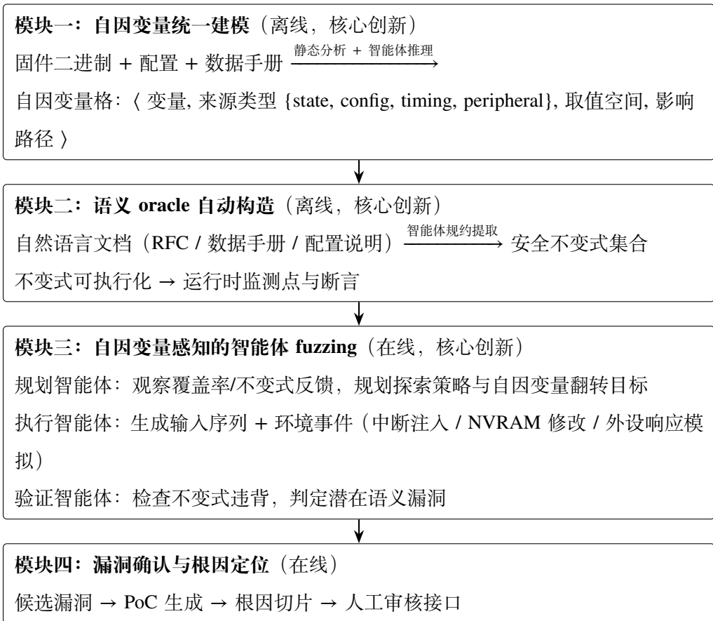
图 3 基于智能体的漏洞挖掘技术路线
