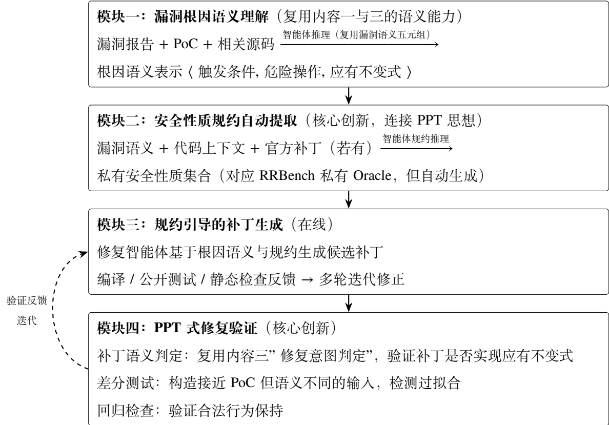
图 3 基于智能体的漏洞自动修复技术路线
