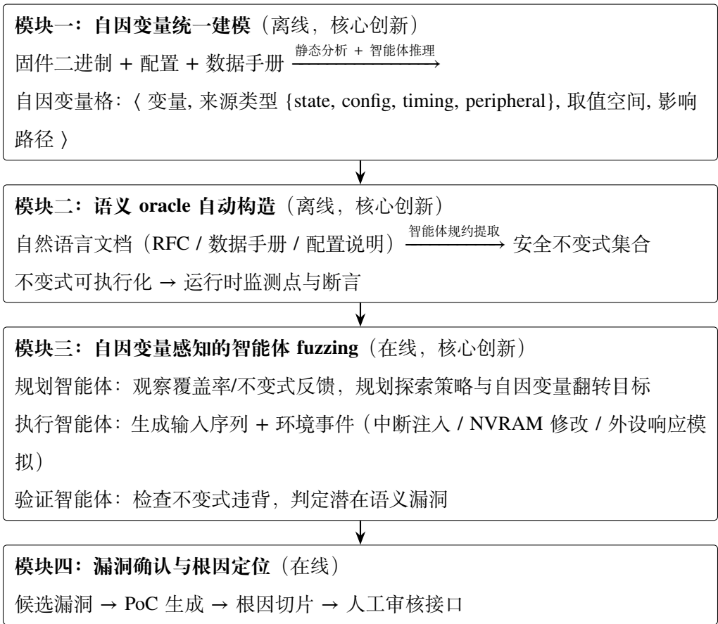
图 2 基于智能体的语义漏洞挖掘技术路线
