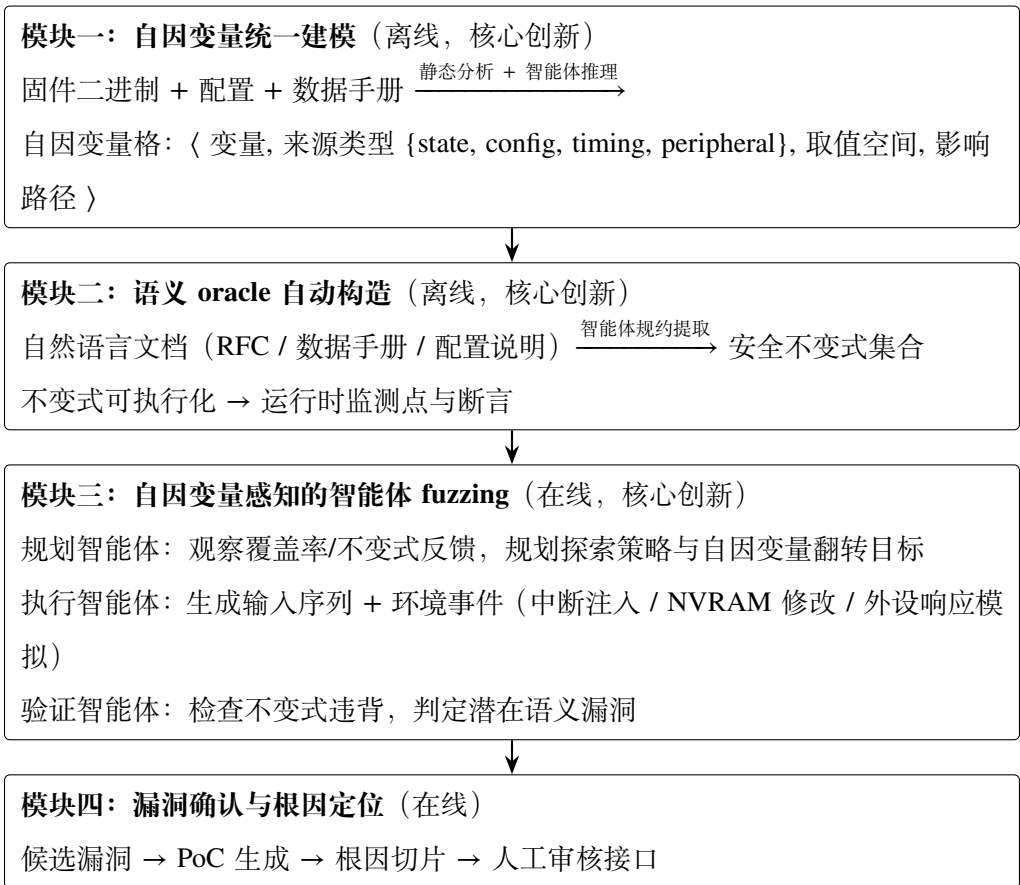
图 2 基于智能体的漏洞挖掘技术路线
