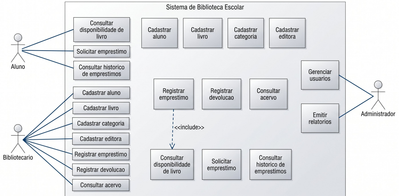
Diagrama de Caso de Uso - Biblioteca Escolar
