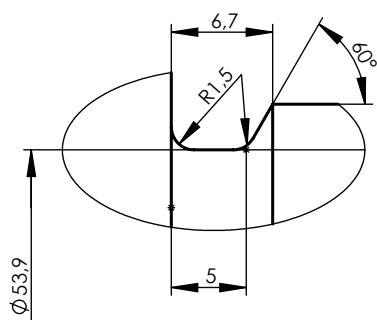
DETTAGLIO X Gola di scarico filettatura SCALA 2 : 1
