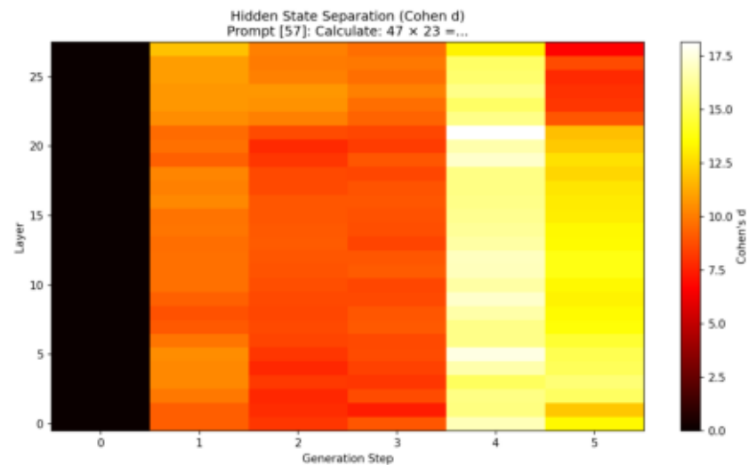
(d) Math
