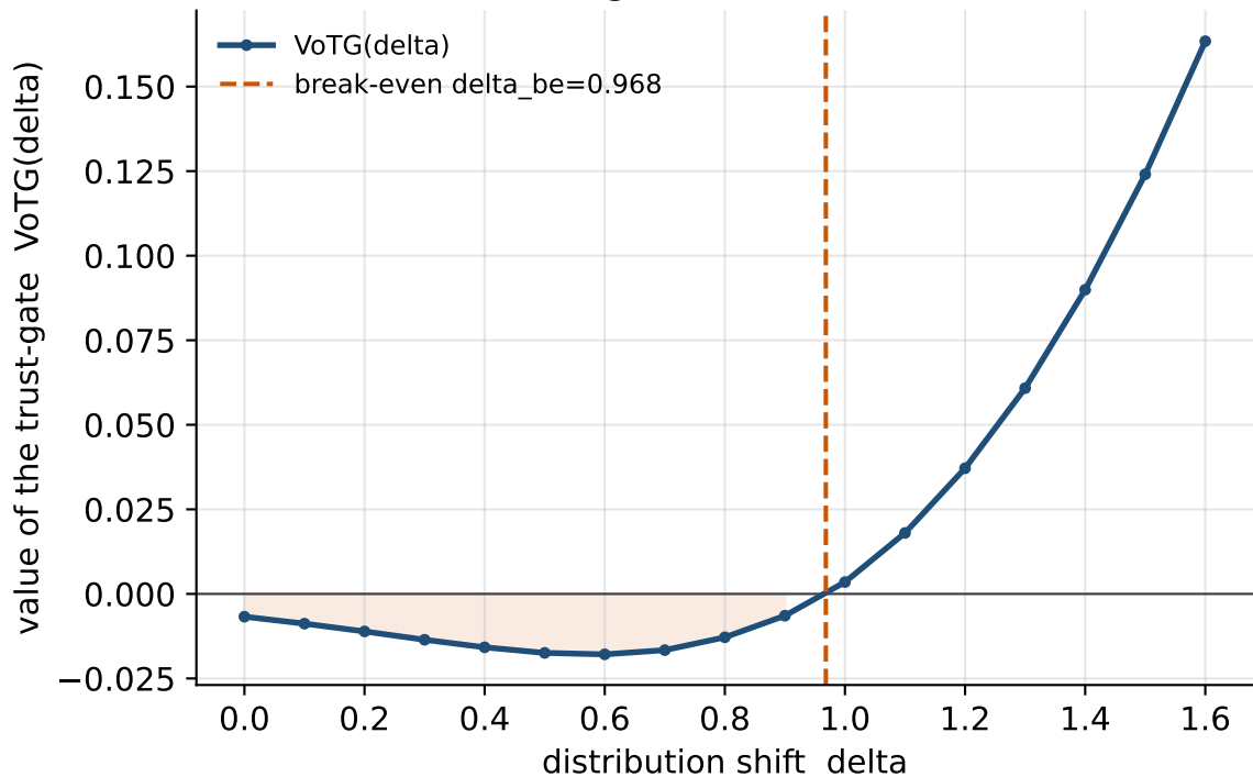
(d) Trust-gate break-even shift
