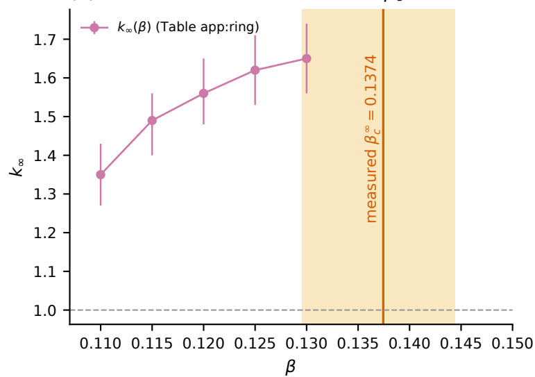
(d) k_\infty rises toward the measured \beta_c
