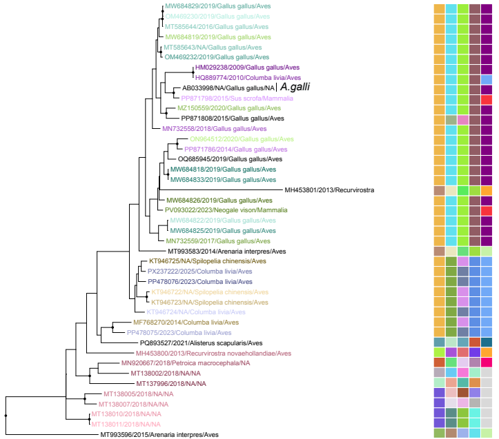
ORF2_2
