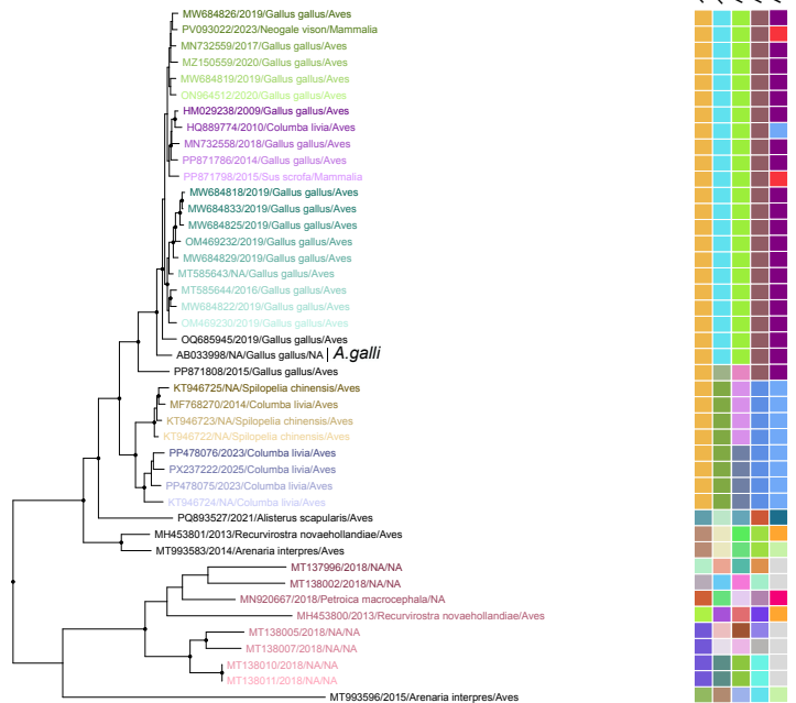
ORF2_2
