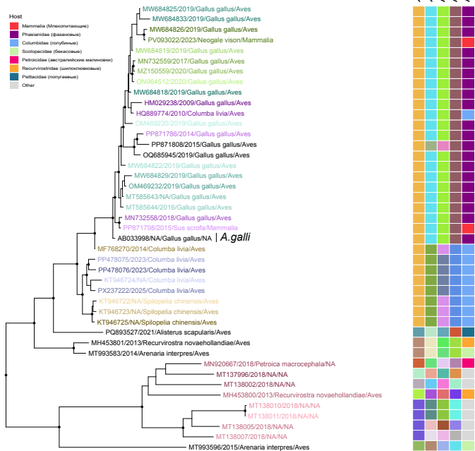
ORF2_1
