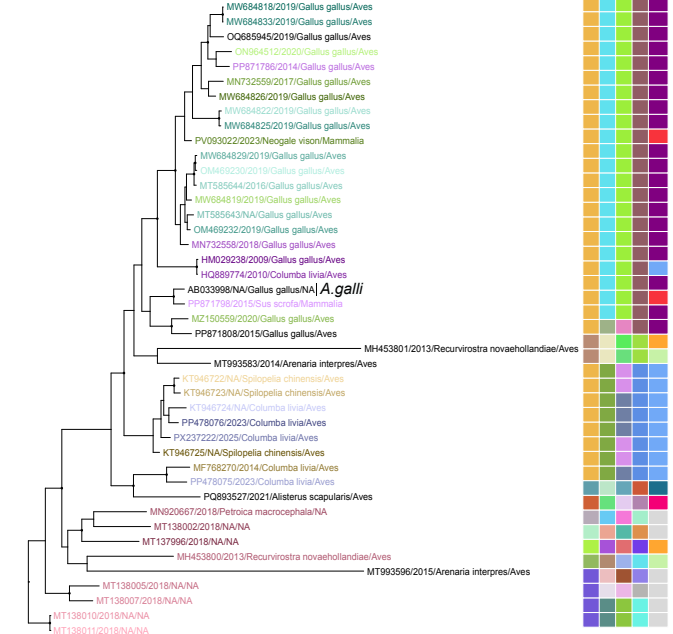
ORF2
