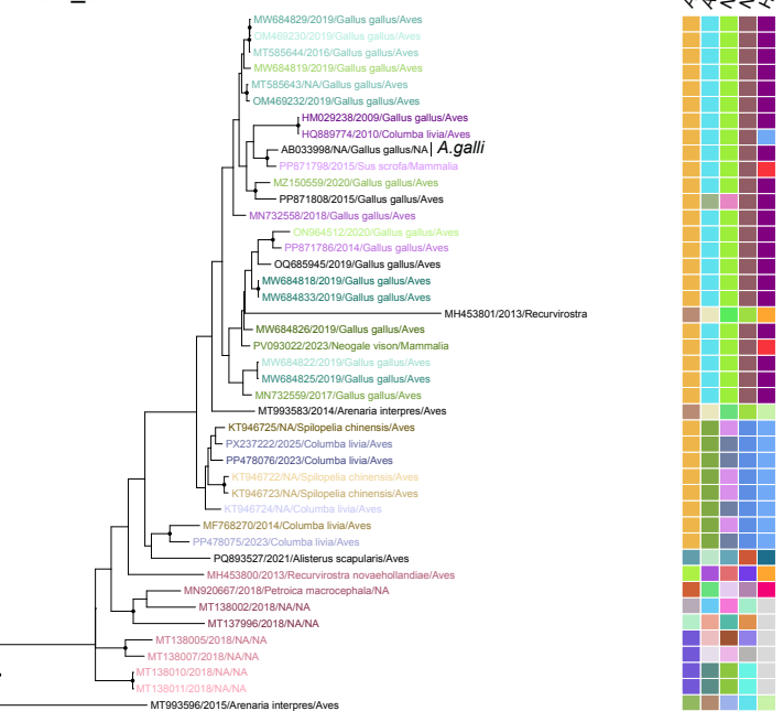
ORF2_2
