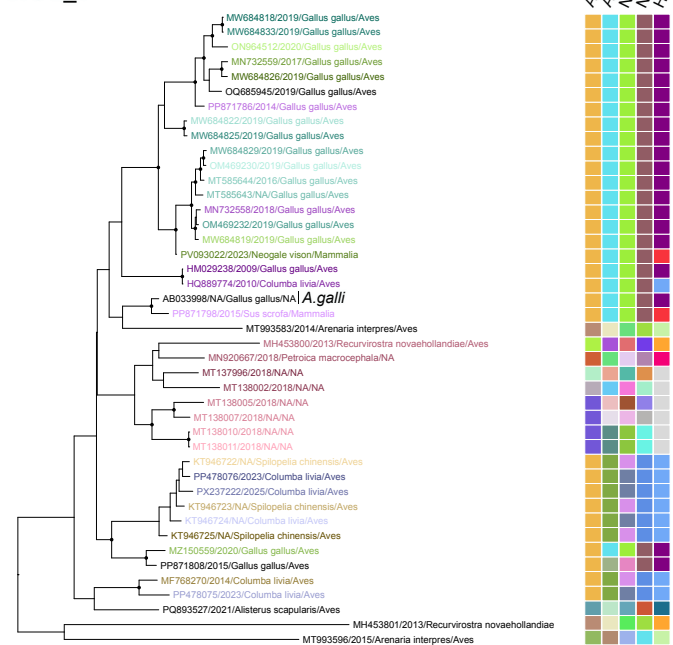
ORF2_1
