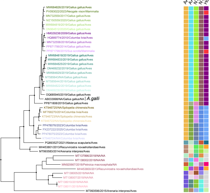
ORF2_2
