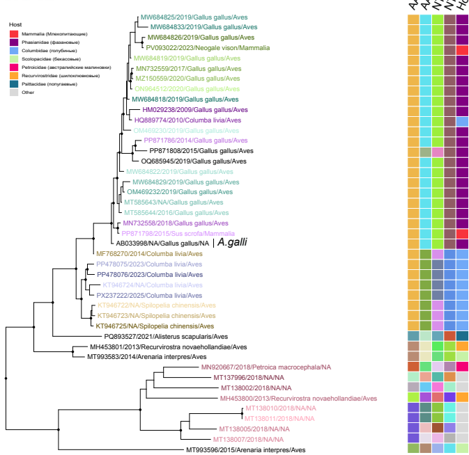
ORF2_1
