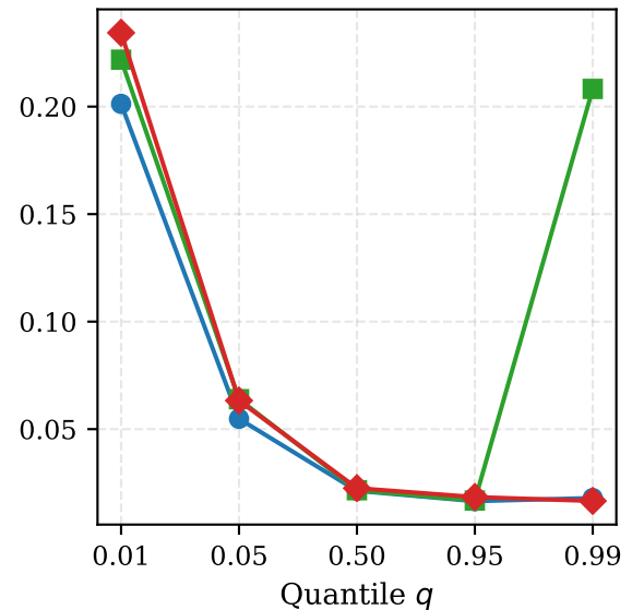
Gumbel
