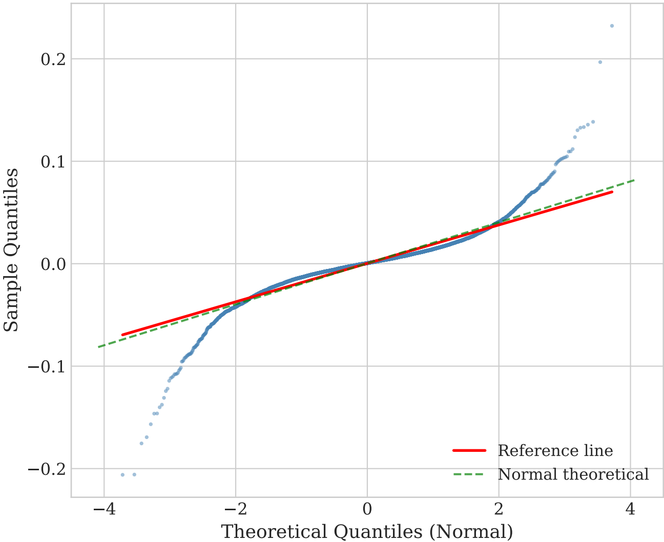
(d) QQ-Plot: Log Returns vs Normal Distribution
