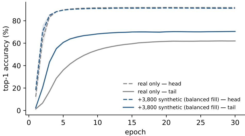
Food101-LT, IR 150
