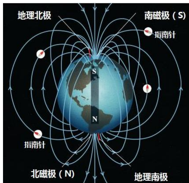
地球磁偶极子场
