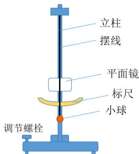
图 2.4-5 单摆实验装置
