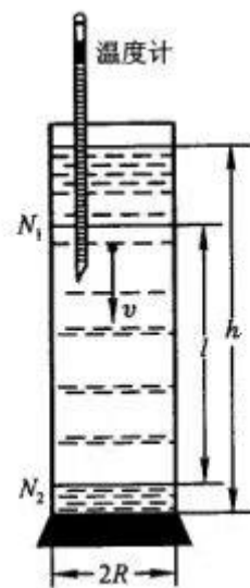
图 2 落球法测定液体的粘度装置图
