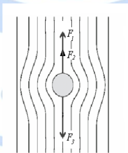
图 1 小球在液体中下落
