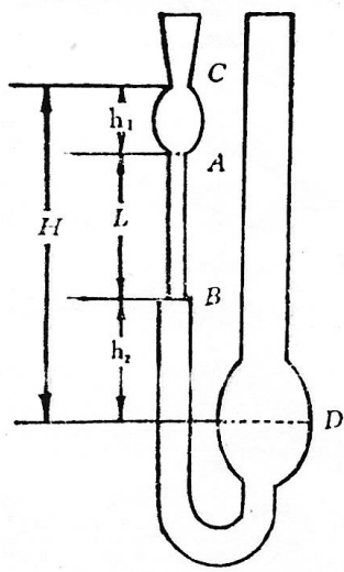
图3 毛细管粘度计
