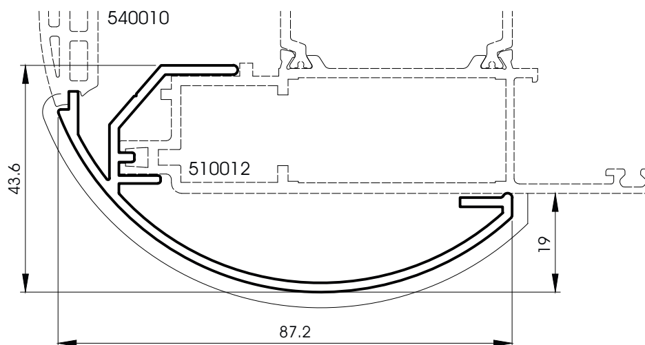
520010 Stile nip-guard
