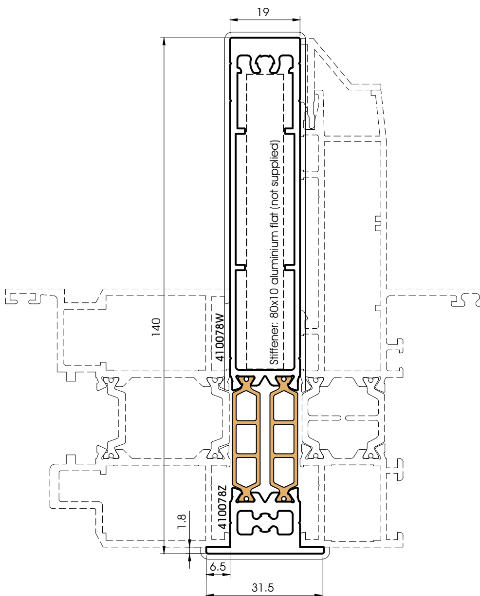
410078 50-70 stiffener
