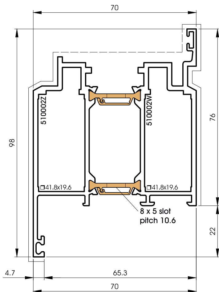
510002 Inward opening
