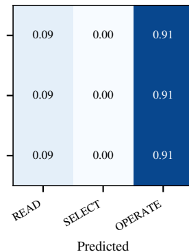
(d) A fixed on Obfuscated, both
