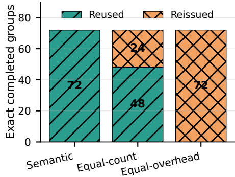
(b) Live LiH: 18 cases
