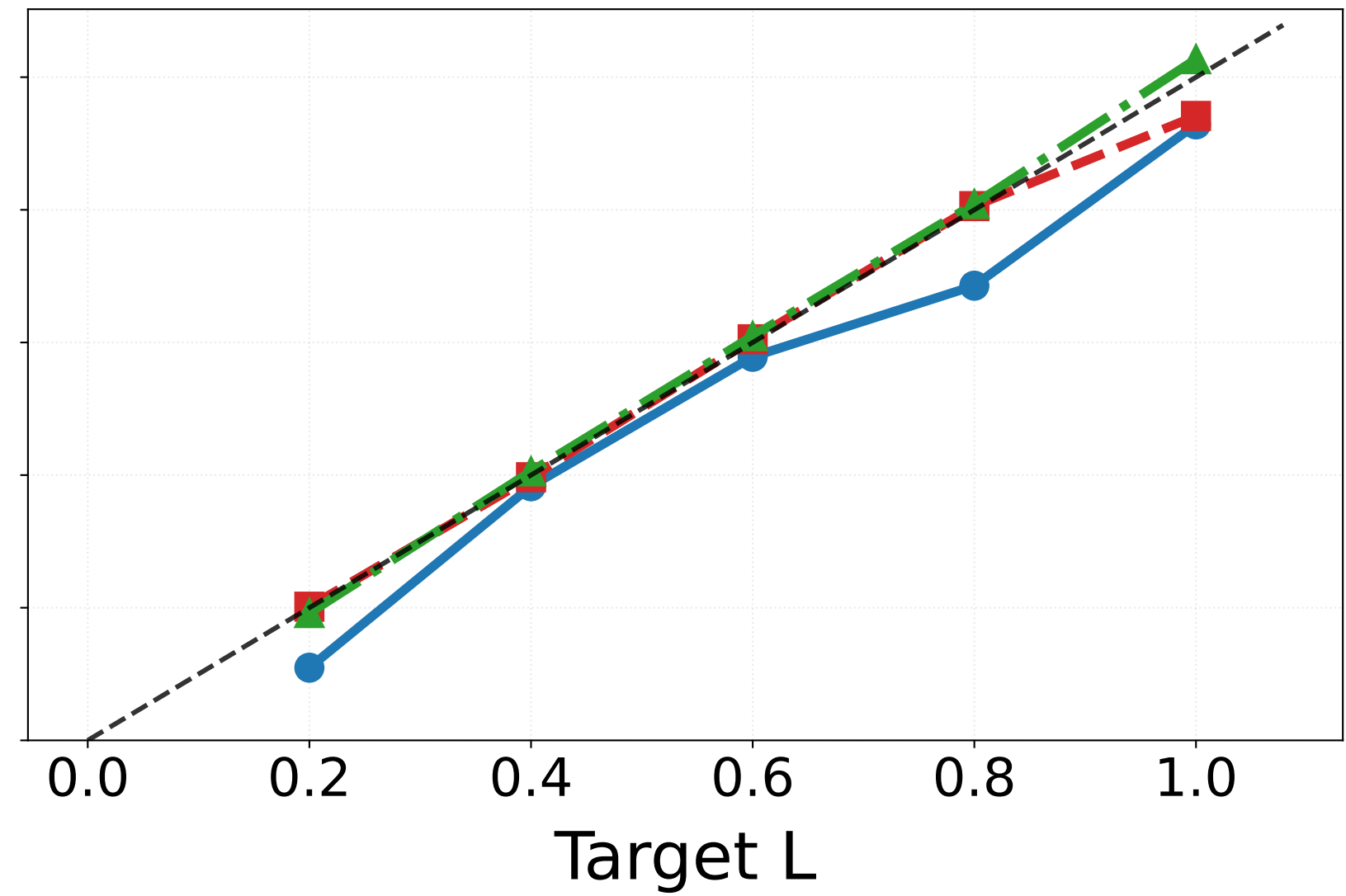
Softmax
