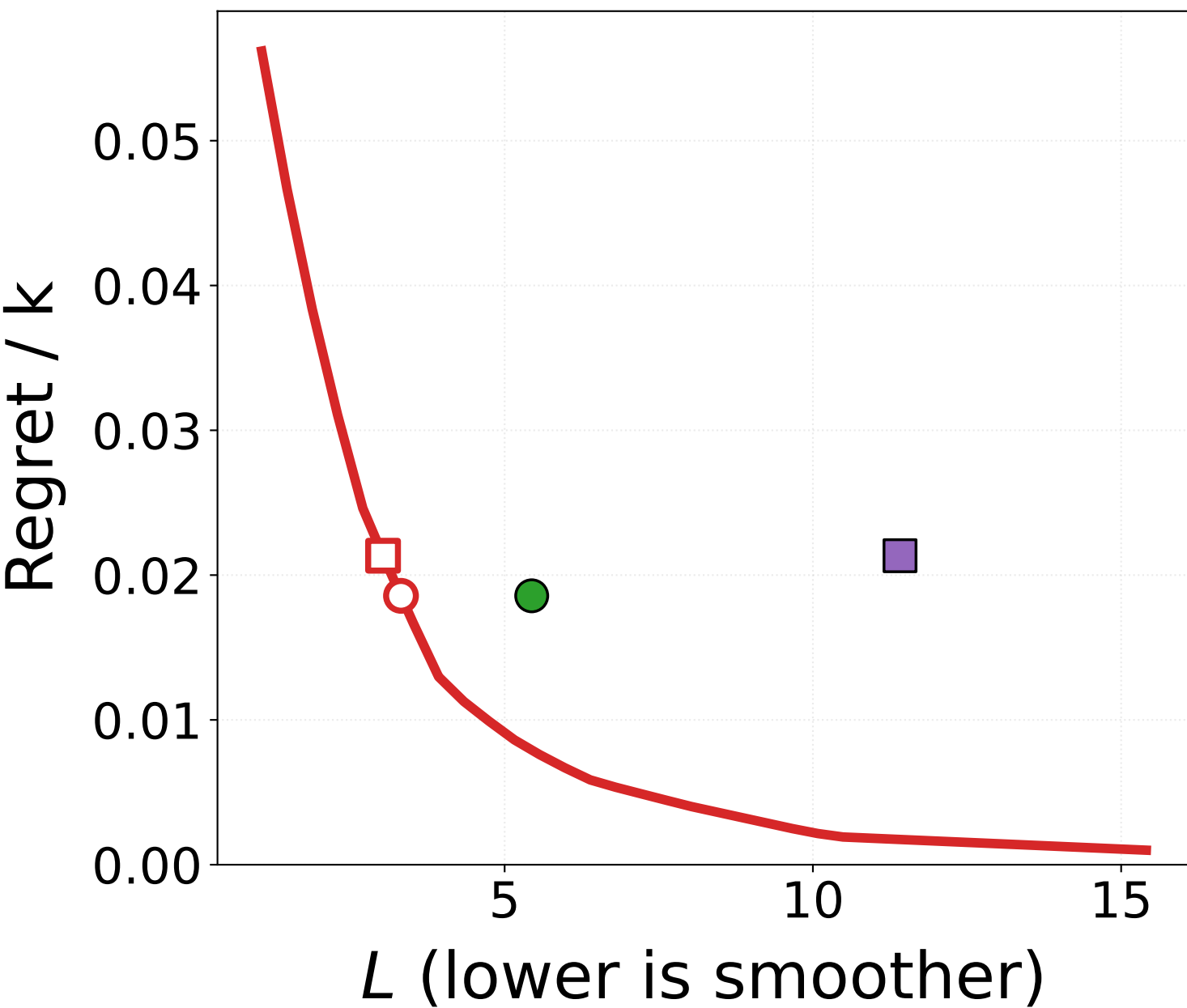
ICLR
