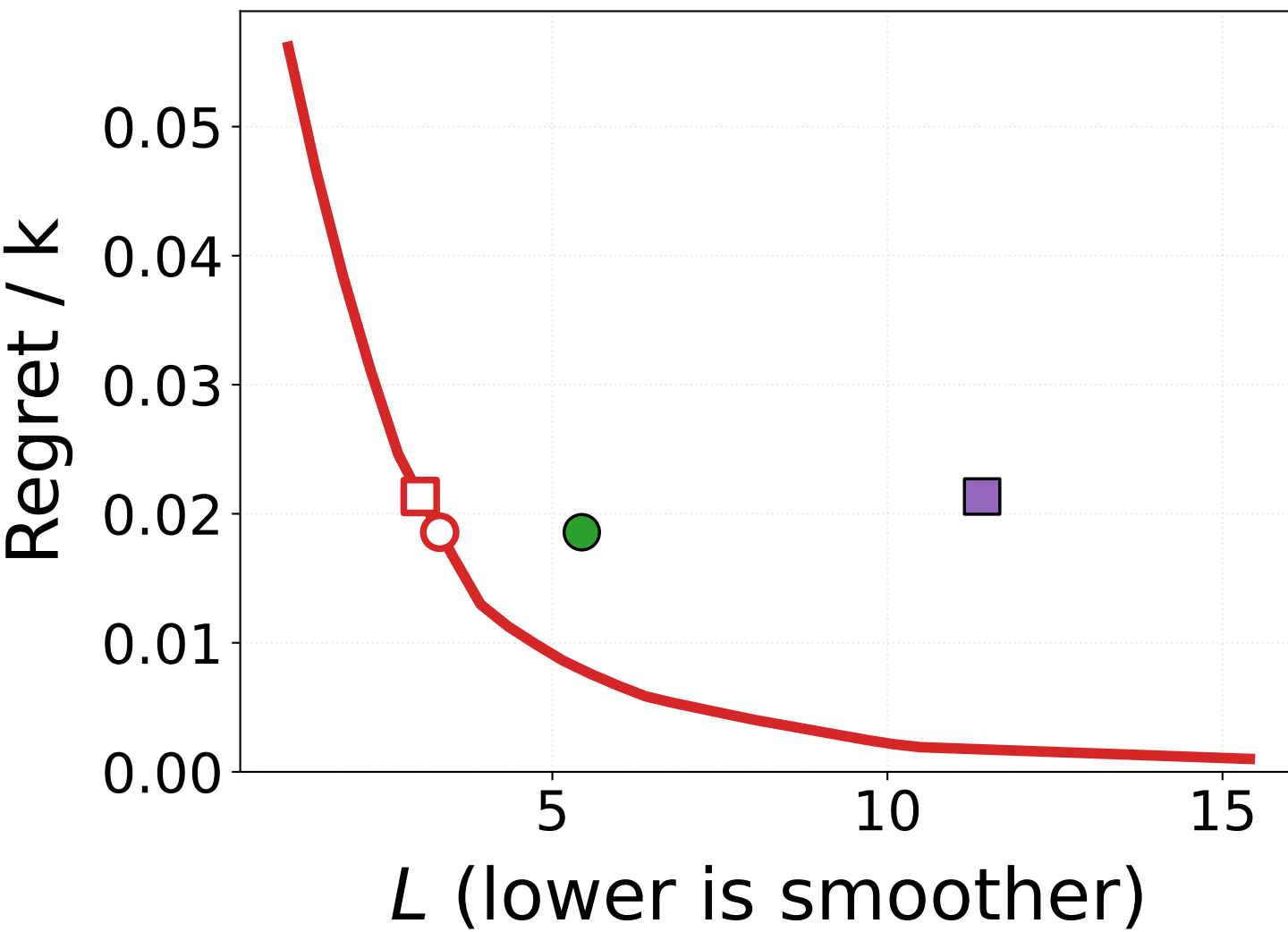
ICLR
