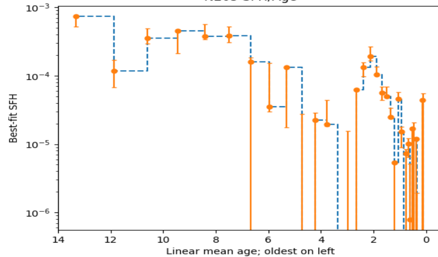
N205 SFH/Age
